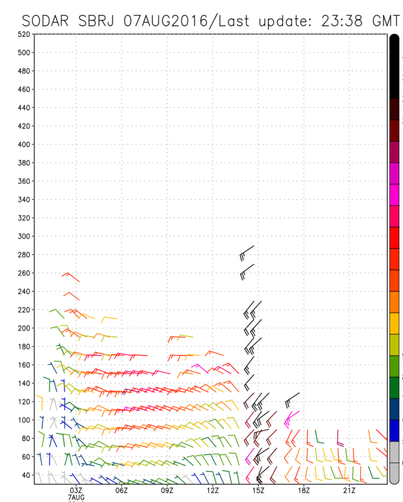
Figura 4 – Dados observacionais de vento horizontal estimados pelo SODAR.
