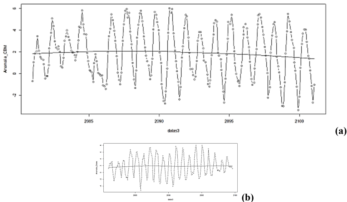
Figura 1 – (a) Anomalia da Temperatura da Superfície do Mar sob influência de aquecimento global para a Região da CBM (b) O mesmo para a Passagem de Drake.
