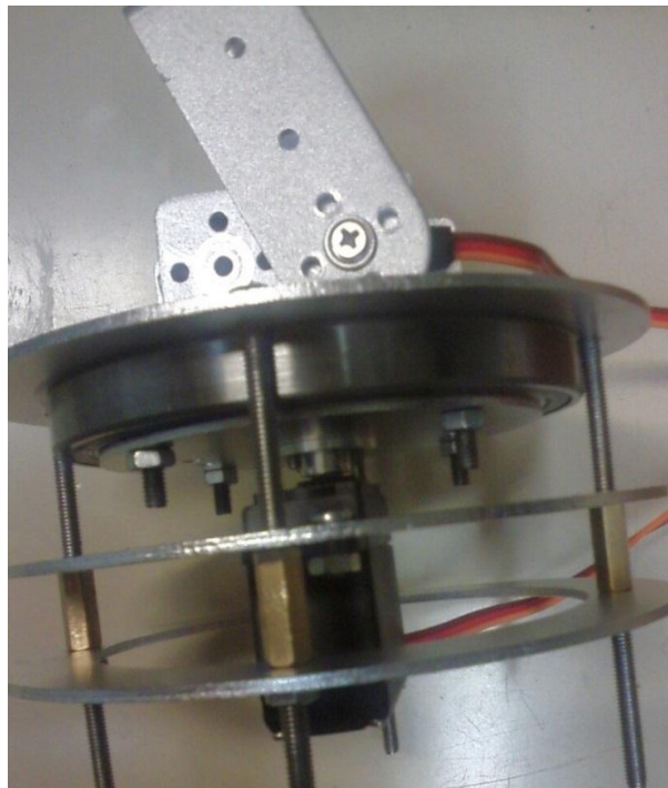
Figura 11 – PAN/TILT de metal (vista lateral)
