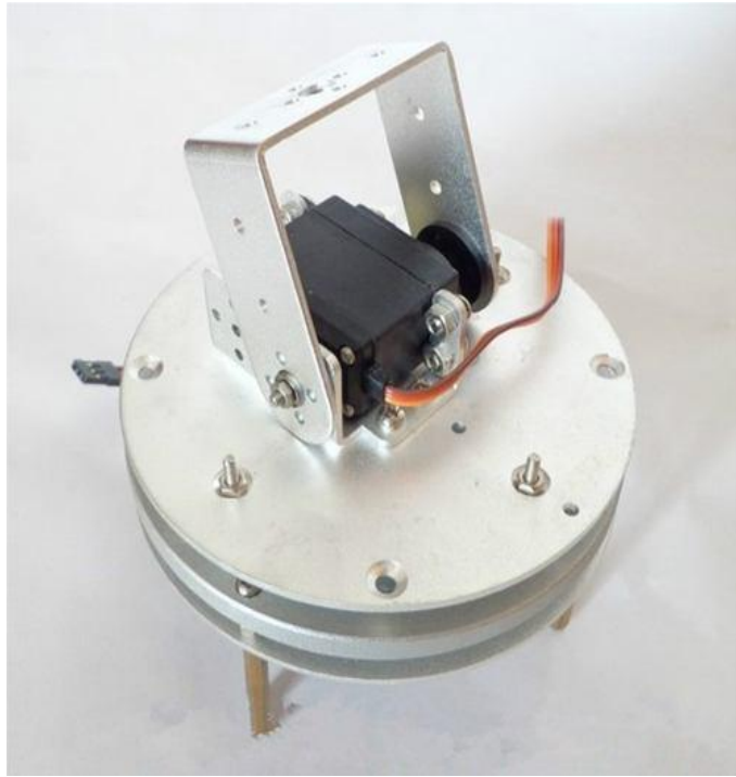
Figura 10 – PAN/TILT de metal (vista superior)
