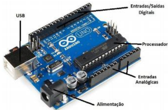
Figura. 5 - Arduino Uno e suas principais partes
