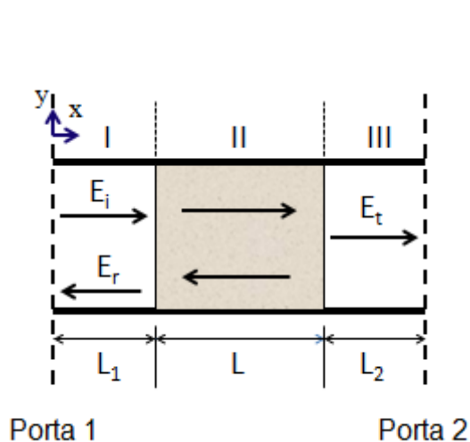
Figura 1. Esquema da estrutura do trecho de guia de onda preenchido com material a ser investigado junto com as ondas incidente, refletida e transmitida.
