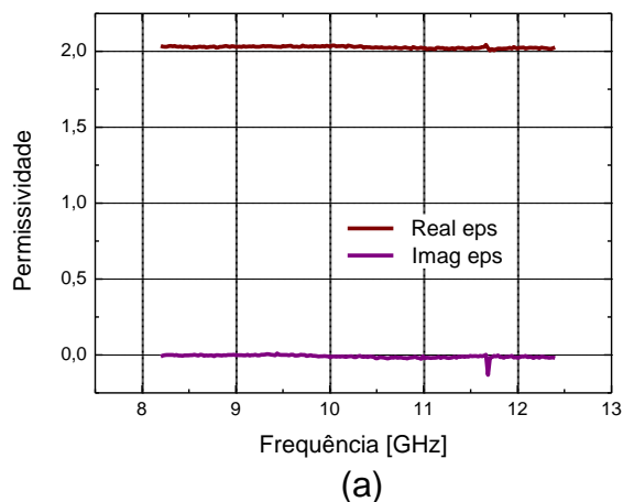
Figura 7. Valores medidos das componentes reais e imaginárias da (a) permissividade (eps) e (b) permeabilidade (mu) em função da frequência para o teflon de 5 mm de espessura.
