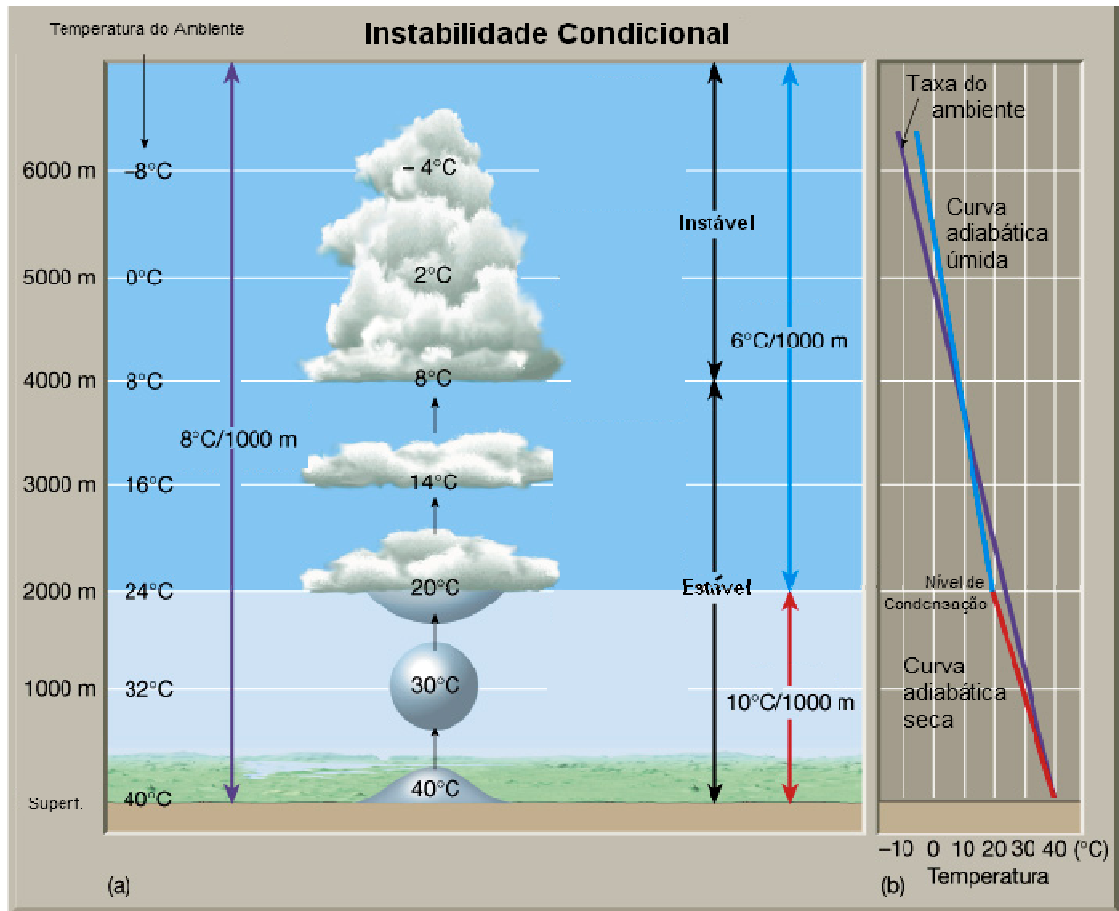
Figura 4.2 – Representação esquemática de uma parcela de ar saturada onde em (a) necessita de uma forçante para superar a estabilidade e em (b) o diagrama termodinâmico representando a instabilidade condicional.
