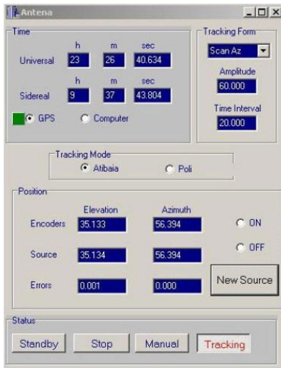
Figura 1 - Configuração da antena e status
