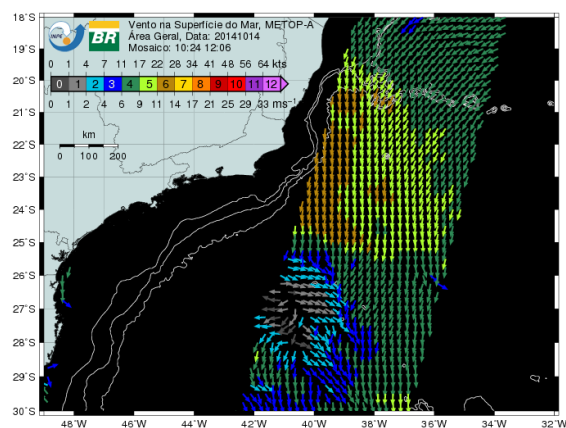
Figura 6: Campo de vento obtido via satélite.
