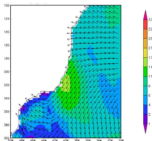
Figura 2: Campo de vento BRAMS
