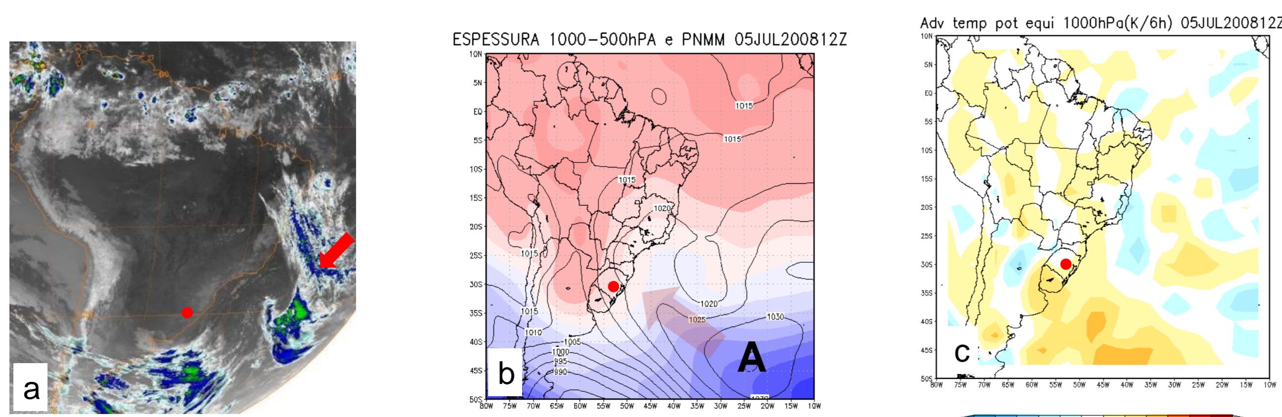
Figura 3- Imagem de satélite no canal IR (a), espessura (b) e adv. θe (c). Fonte: NOAA.
