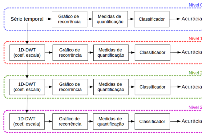
Figura 3: Fluxo da metodologia proposta.
