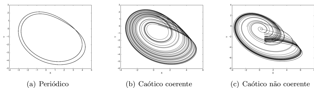
Figura 4: Diferentes comportamentos presentes no sistema de Rössler.
