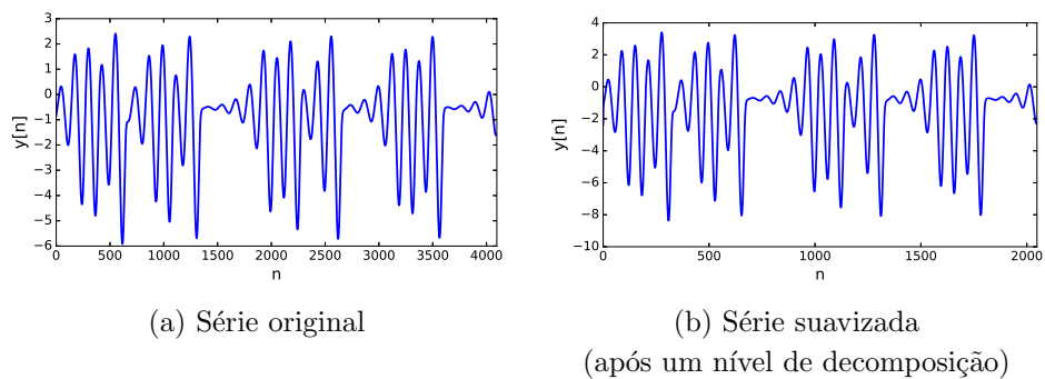
Figura 1: Exemplo da aplicação da transformada wavelet discreta. Nesse exemplo, usou-se a wavelet ortogonal de Daubechies com ordem 4 de aproximação local com um nível de decomposição.
