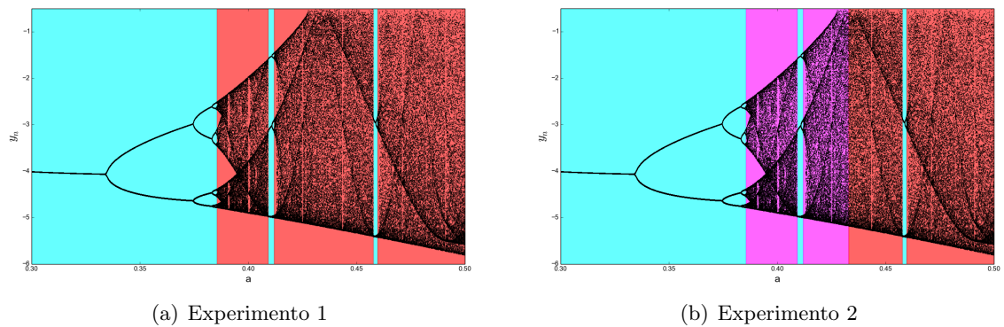
Figura 5: Localização das regiões caótica e não caótica do sistema de Rössler.
