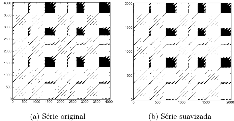
Figura 2: Gráficos de recorrência das séries temporais da Figura 1. Nessa representação, pontos pretos e brancos representam estados recorrentes e não recorrentes, respectivamente.
