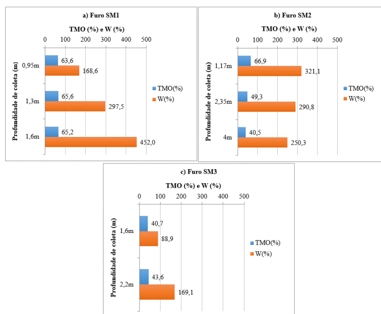
Figura 2 – Teor de umidade gravimétrico W (%) e teor de matéria orgânica (TMO) como função da profundidade para as amostras secas ao ar.
