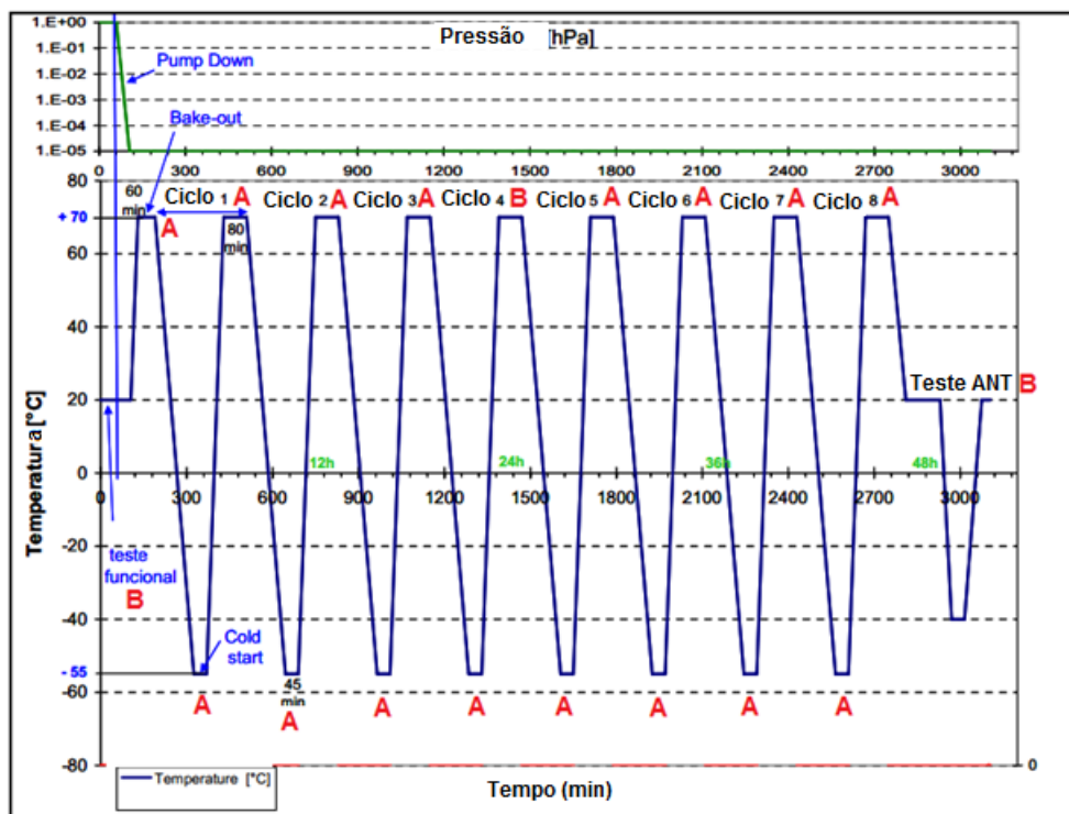
Figura 6-5: Perfil de temperaturas, vácuo e testes funcionais.
