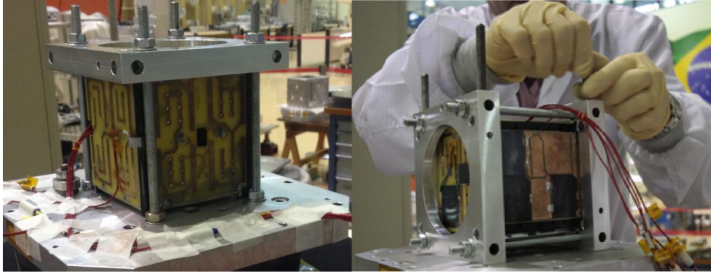
Figura 6-3: Montagem vertical e horizontal respectivamente da interface Test-POD14 com o AESP14 – QM.
