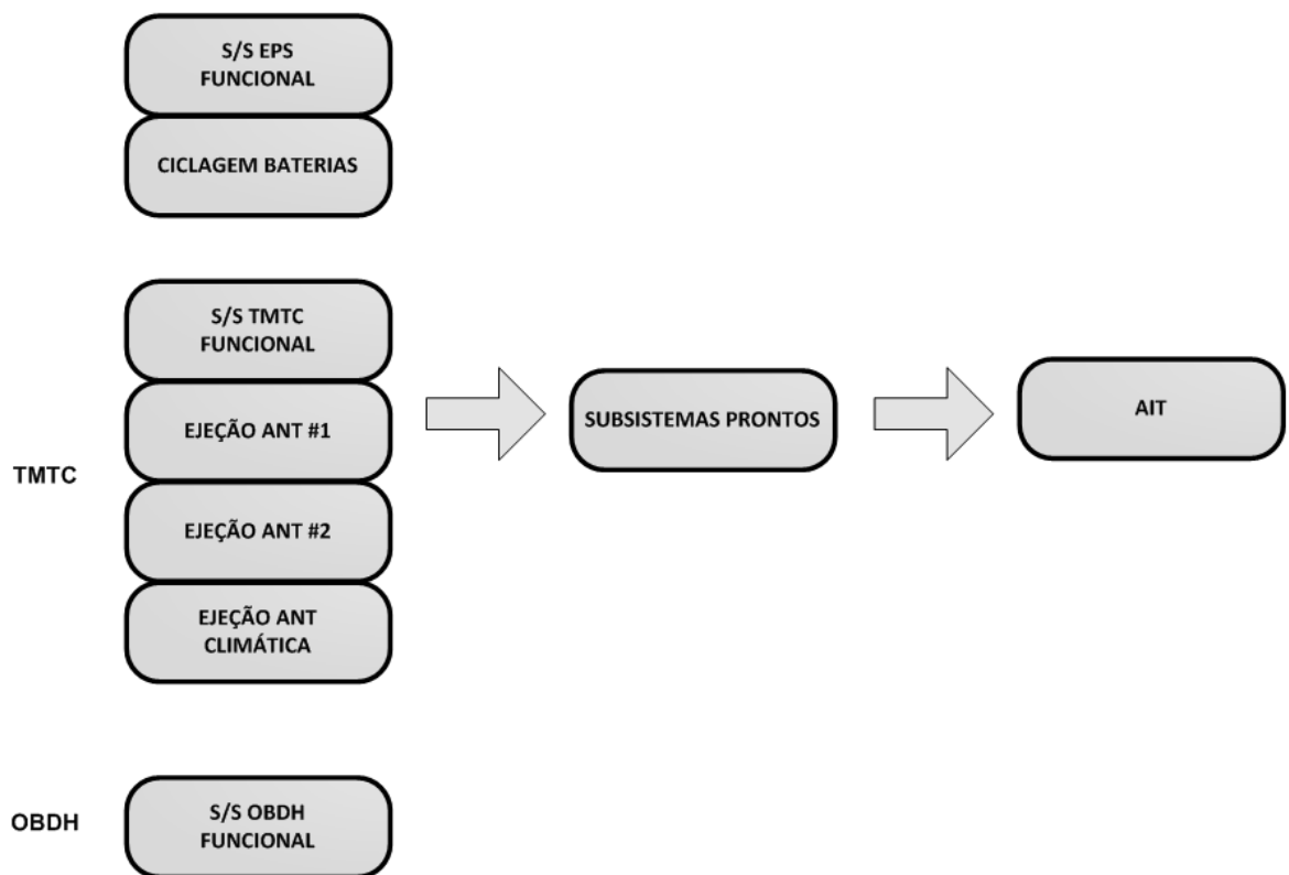
Figura 7-1: Testes de subsistema - QM.
