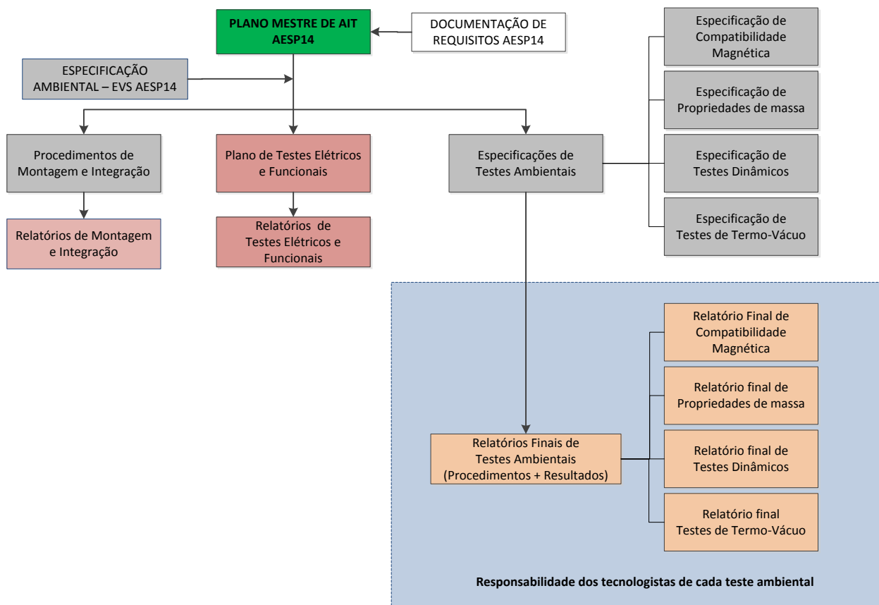
Figura 4-1: Estrutura geral da documentação de AIT do AESP14.
