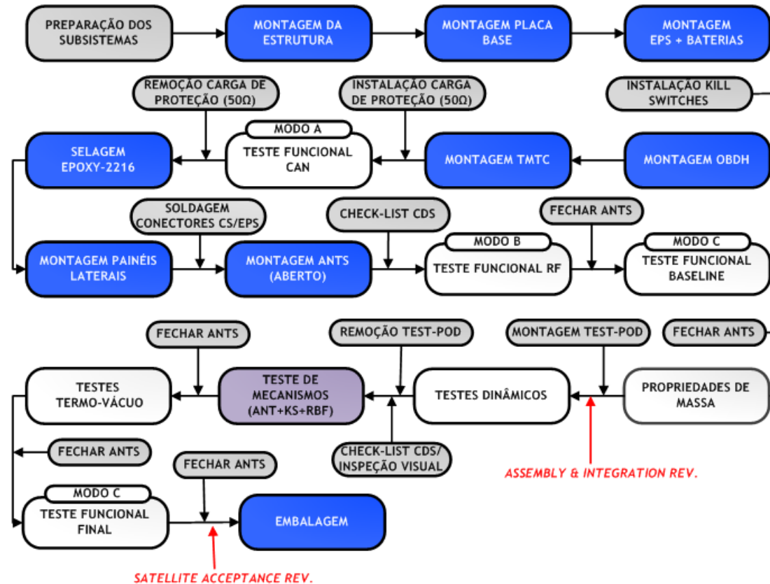
Figura 4-8: Sequência de montagem e integração do sistema.
