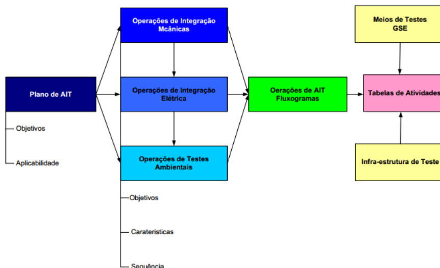
Figura 4.8 - Estrutura do plano de AIT de programas espaciais.
