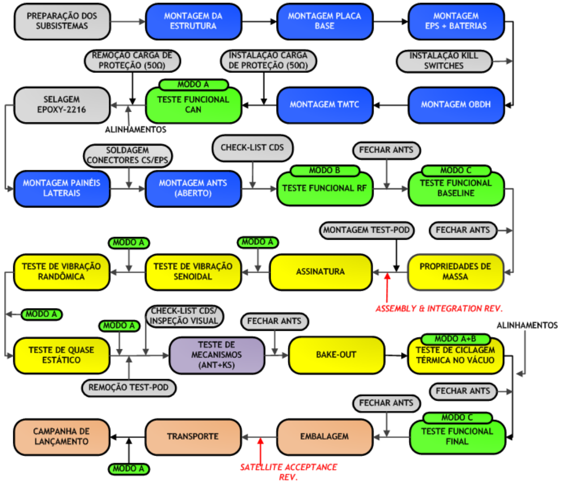
Figura 9-9: Sequência detalhada de AIT do FM.
