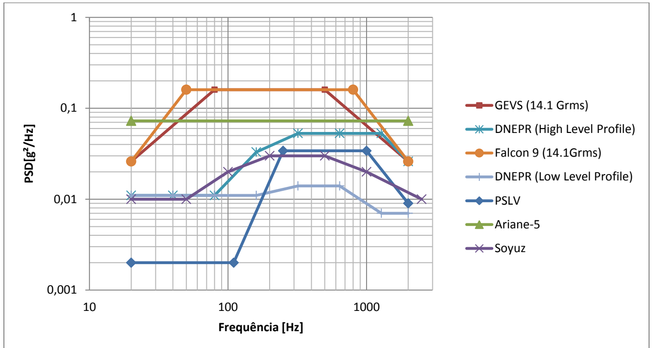
Figura 4-2: Níveis de teste para ensaio randômico.
