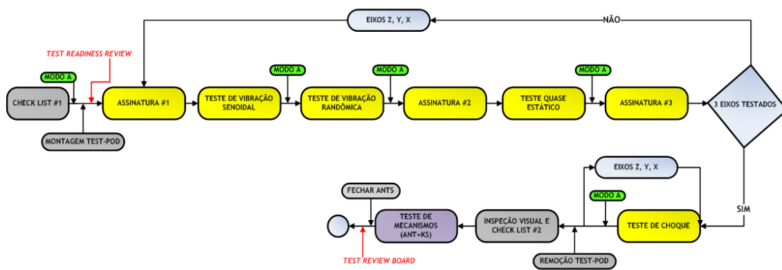
Figura 4.19 - Sequência detalhada de Testes dinâmicos.
