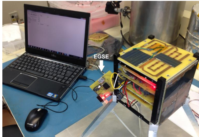
Figura 6-5: EGSE para verificação funcional do AESP14 – QM.
