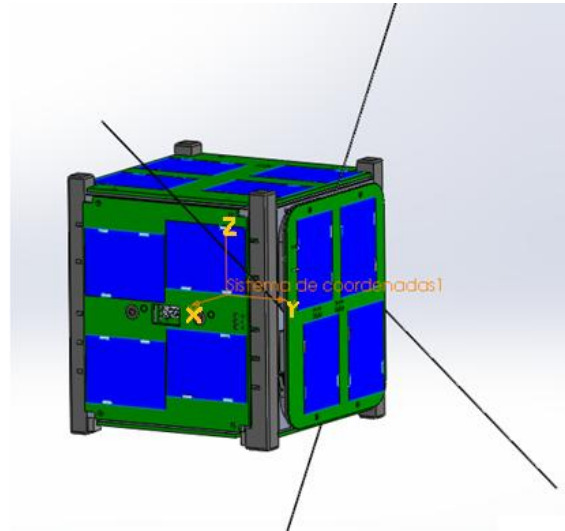
Figura 4-1: Sistema de coordenadas adotado pelo Projeto.
