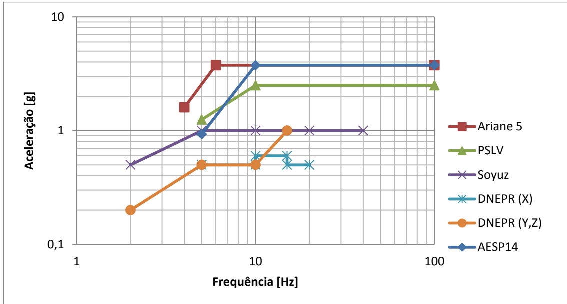
Figura 4-1: Níveis de teste para ensaio senoidal.
