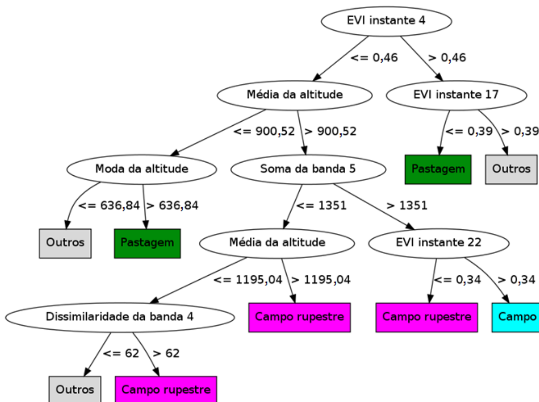
Figura 6.1 Árvore de decisão para o Experimento 1 (EVI + Landsat + TOPODATA).
