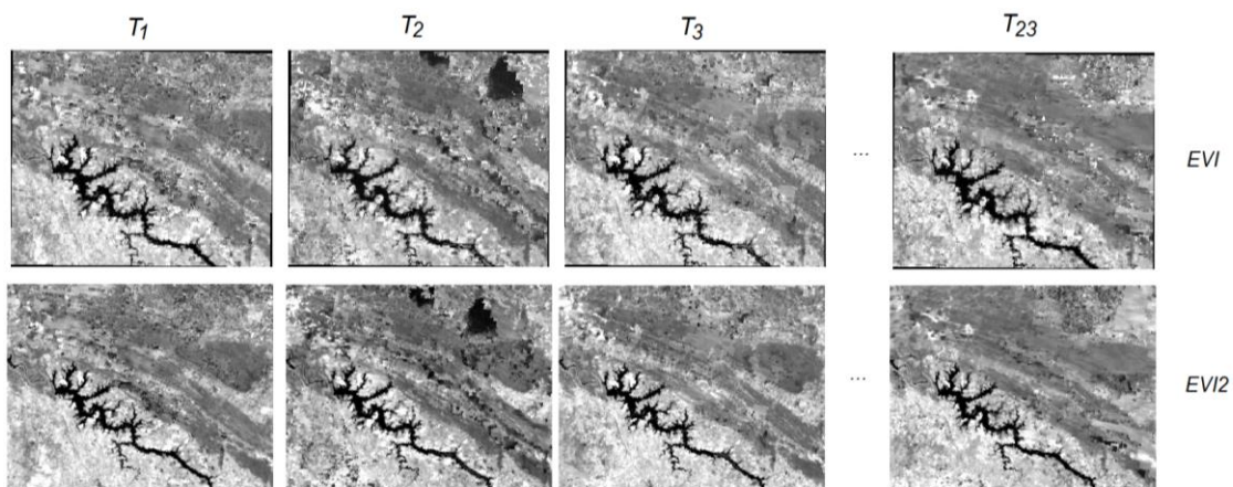
Figura 5.7 Sequência de imagens para compor os perfis anuais de EVI e EVI2 para o ano de 2009.
