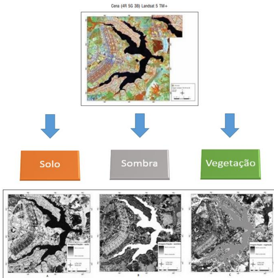
Figura 3.4. Exemplo da aplicação do MLME e suas imagens-fração resultantes.
