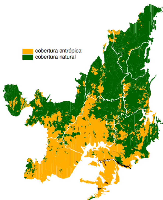
Figura 5.4 Regiões do Cerrado mapeadas pelo MMA como áreas naturais (em verde) e antrópicas (em amarelo).
