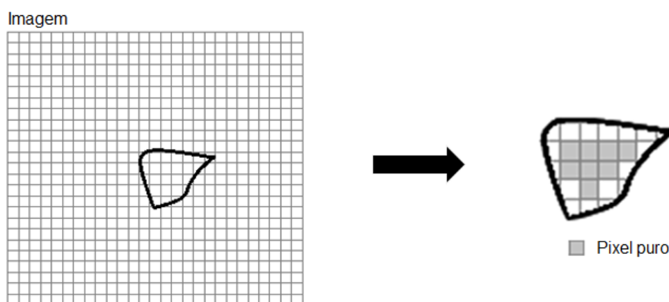
Figura 5.9 Abordagem de pixels puros.
