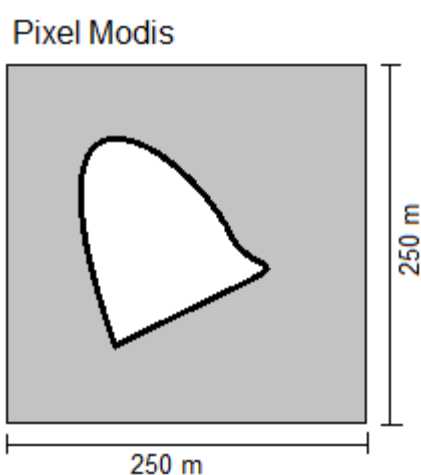
Figura 5.10 Exemplo de polígono desconsiderado do conjunto de amostras na abordagem de pixels puros.
