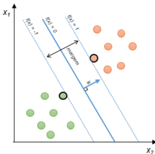
Figura 4.5. Representação do hiperplano ótimo e dos vetores de suporte.
