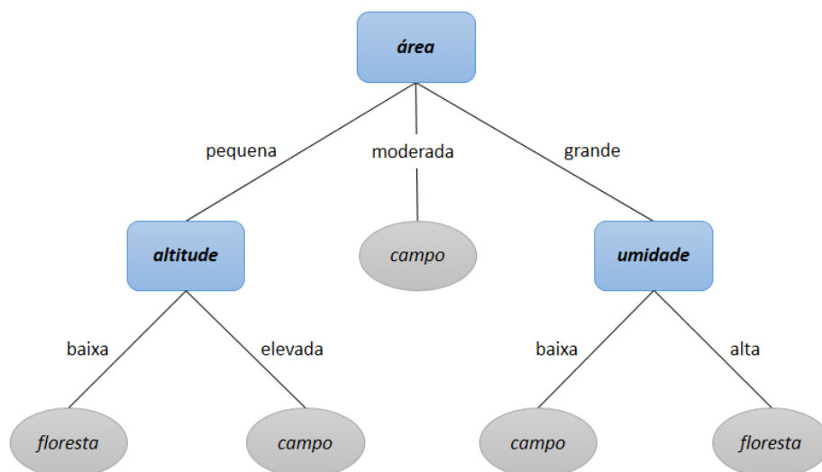
Figura 4.2. Exemplo de árvore de decisão indicando se uma região é uma provável floresta ou um campo.
