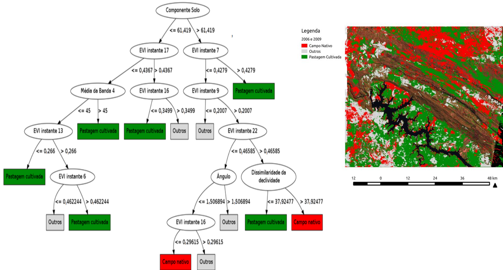
Figura 6.2. Árvore de decisão (à esquerda) e mapeamento (à direita) para o melhor resultado encontrado no Experimento 3.
