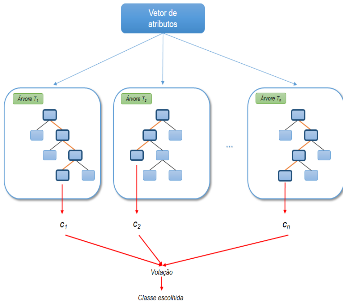
Figura 4.3. Exemplo do processo de seleção de uma classe a partir da classificação em floresta aleatória.
