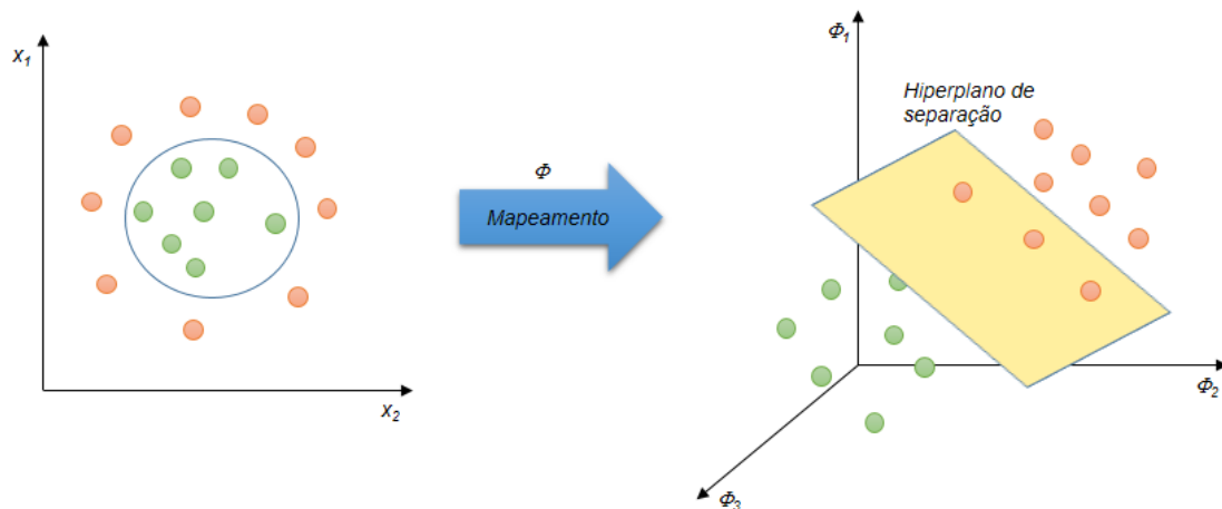
Figura 4.6. Exemplo de mapeamento para um espaço de maior dimensão, fornecendo uma separação linear.
