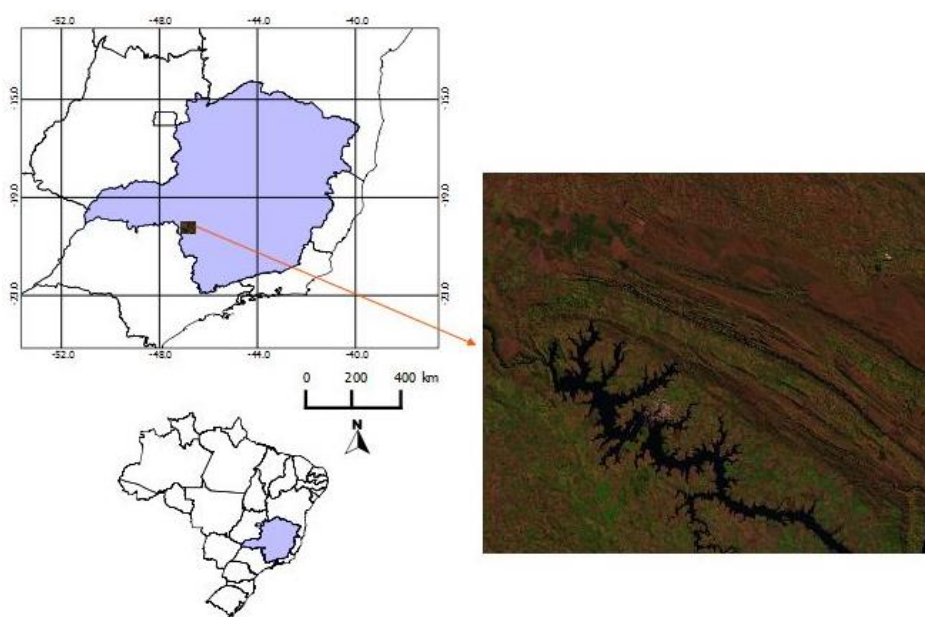
Figura 5.1 Área de estudo do trabalho, localizada no sudoeste do estado de Minas Gerais. Recorte de uma imagem Landsat TM-5 (R5B4G3) da região.
