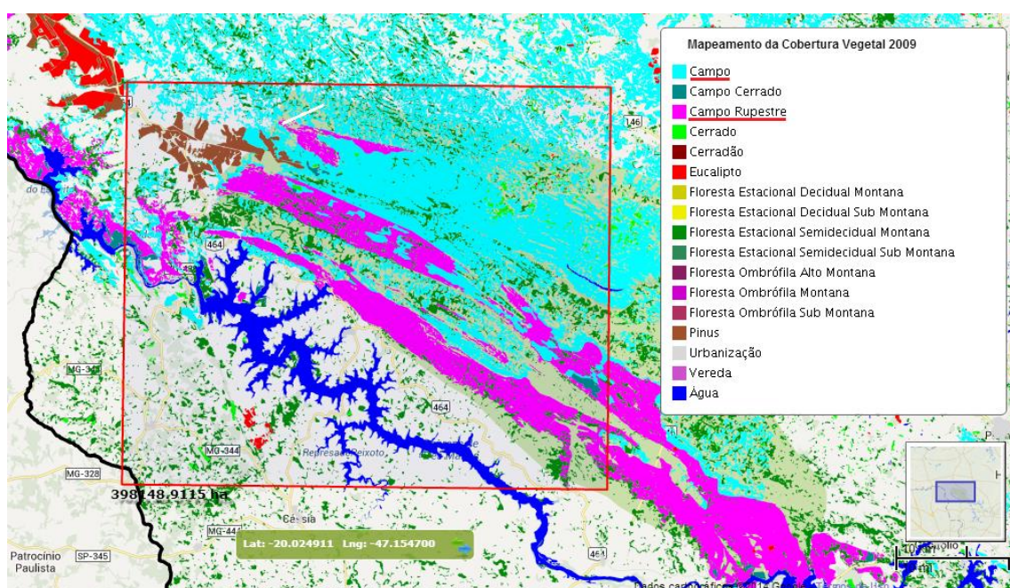
Figura 5.3 Mapa de referência utilizado na área de estudo para obtenção das regiões de formações campestres: Campo (cor ciano) e Campo Rupestre (cor rosa).
