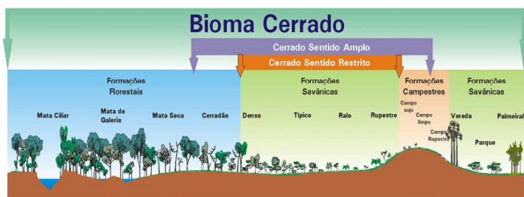
Figura 2.2. Fitofisionomias do bioma Cerrado.
