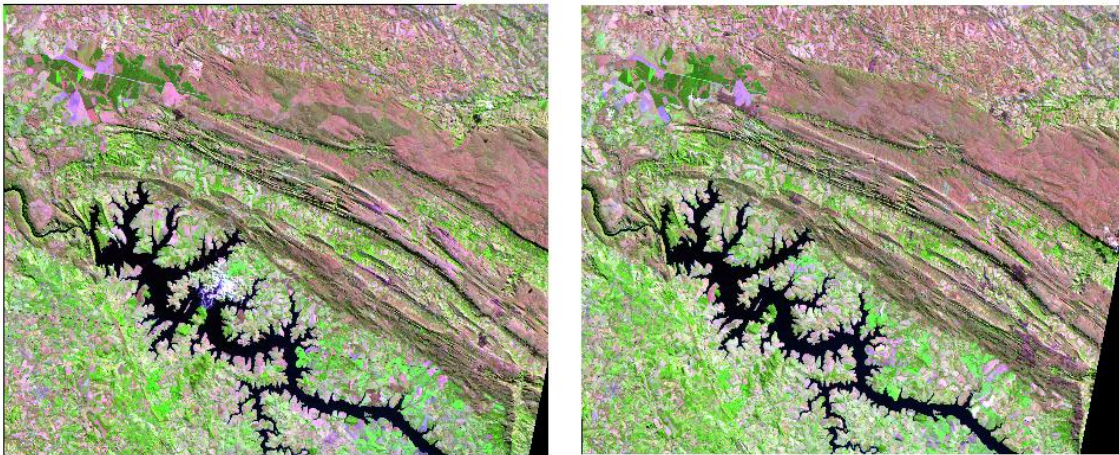
Figura 5.6 Imagens Landsat TM-5 (R5B4G3) de 2006 (esquerda) e 2009 (direita).
