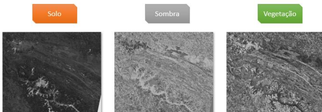
Figura 5.8 Componentes do MLME relativos ao ano de 2006.
