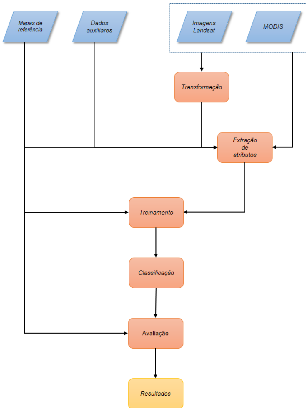
Figura 5.2 Etapas de processamento e análise dos dados.
