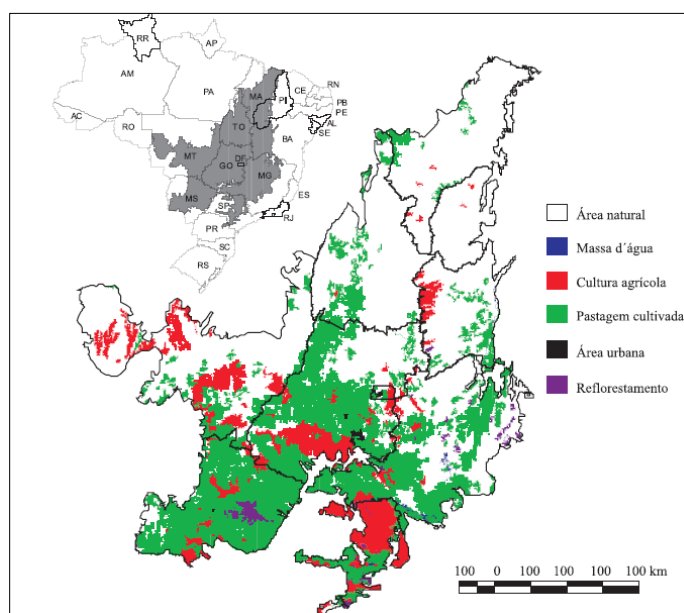
Figura 1.1 Distribuição espacial das classes de uso da terra no bioma Cerrado referente ao ano de 2002.
