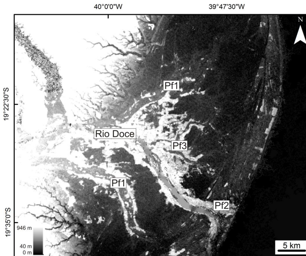
Figura 7.13 – Indicação das três fases representativas dos paleocanais do delta do rio Doce e do curso atual desse rio identificados no MDE-SRTM. Observar os dois paleocanais correspondentes à fase 1, situados a norte (Pf1) e a sul (Pf1) do rio Doce atual, o paleocanal representativo da fase 2 (Pf2) e alguns dos paleocanais da fase 3 localizados a norte do rio Doce (Pf3).
