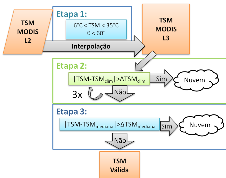
Figura 4.3: Fluxograma do pré-processamento da TSM_{MODIS} (ver detalhes e siglas no texto).
