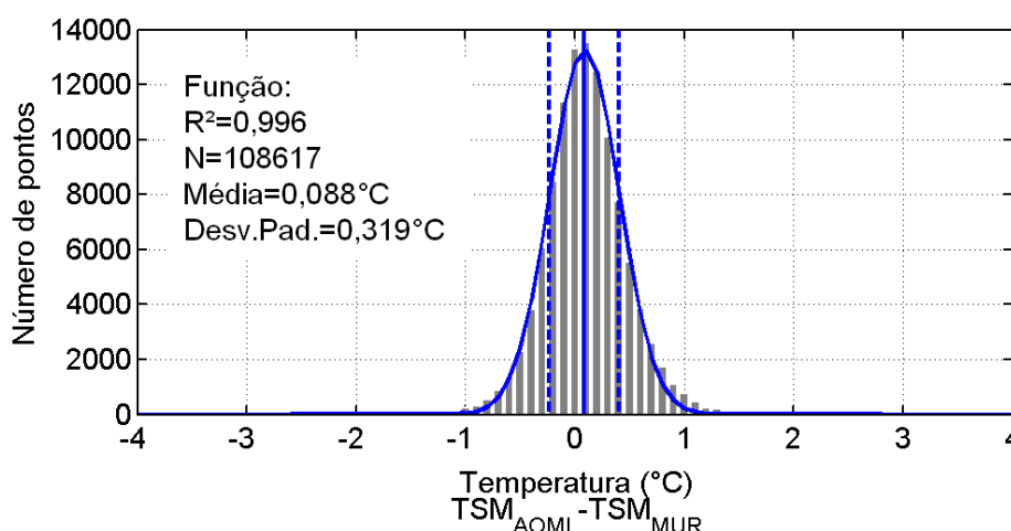
Figura 5.5: Histograma de diferenças (em cinza) entre a TSM_{AOML} e a TSM_{MUR} , em intervalos de 0,1^{\circ}\text{C} . A curva azul representa o ajuste de uma função gaussiana, enquanto as retas verticais representam a média (linha contínua) e um desvio padrão (linha pontilhada) para a função.
