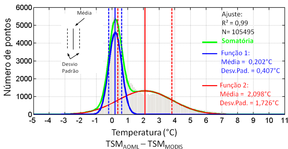
Figura 5.3: Histograma de diferenças entre a temperatura dos derivadores e a TSM_{MODIS} , em intervalos de 0,1^\circ\text{C} (em cinza). As curvas azul e vermelha representam ajustes de duas funções gaussianas e a curva verde representa a somatória das duas. As retas verticais representam a média (linha contínua) e um desvio padrão (linha pontilhada) para cada função.
