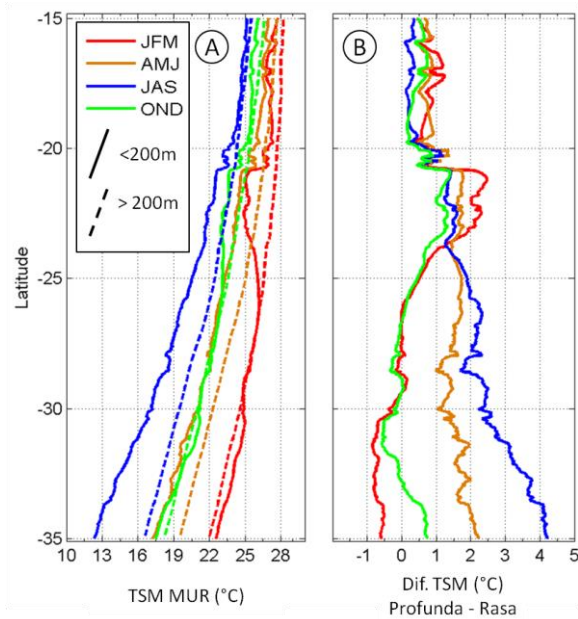
Figura 5.14: Médias zonais da climatologia sazonal da TSM_{MUR} . (A) As linhas contínuas representam a TSM sobre a plataforma (profundidades menor que 200m) e as linhas tracejadas, da região profunda (maior que 200m). (B) Diferença entre as TSM rasa e profunda.
