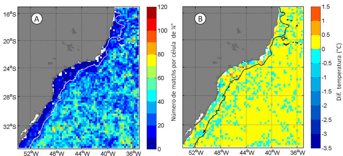
Figura 5.4: Distribuição espacial em grades de 0,25^{\circ} : (A) dos pontos de match-up AOML e MUR e (B) das diferenças médias de TSM_{AOML}-TSM_{MUR} , em ^{\circ}\text{C} . A isóbata representada é de 200m.
