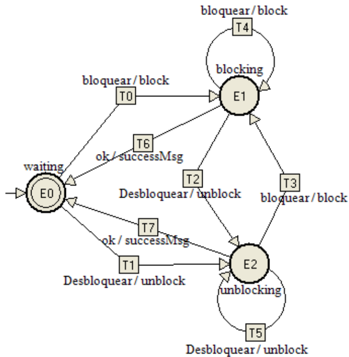
Figura 9 – MEF dos serviços de bloqueio e desbloqueio de acesso, Caso 2.
