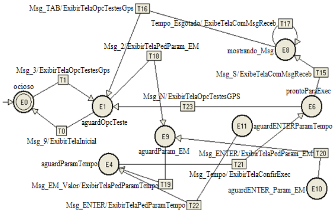
Figura 16 – MEF do serviço Elevation Mask, Caso 4.
