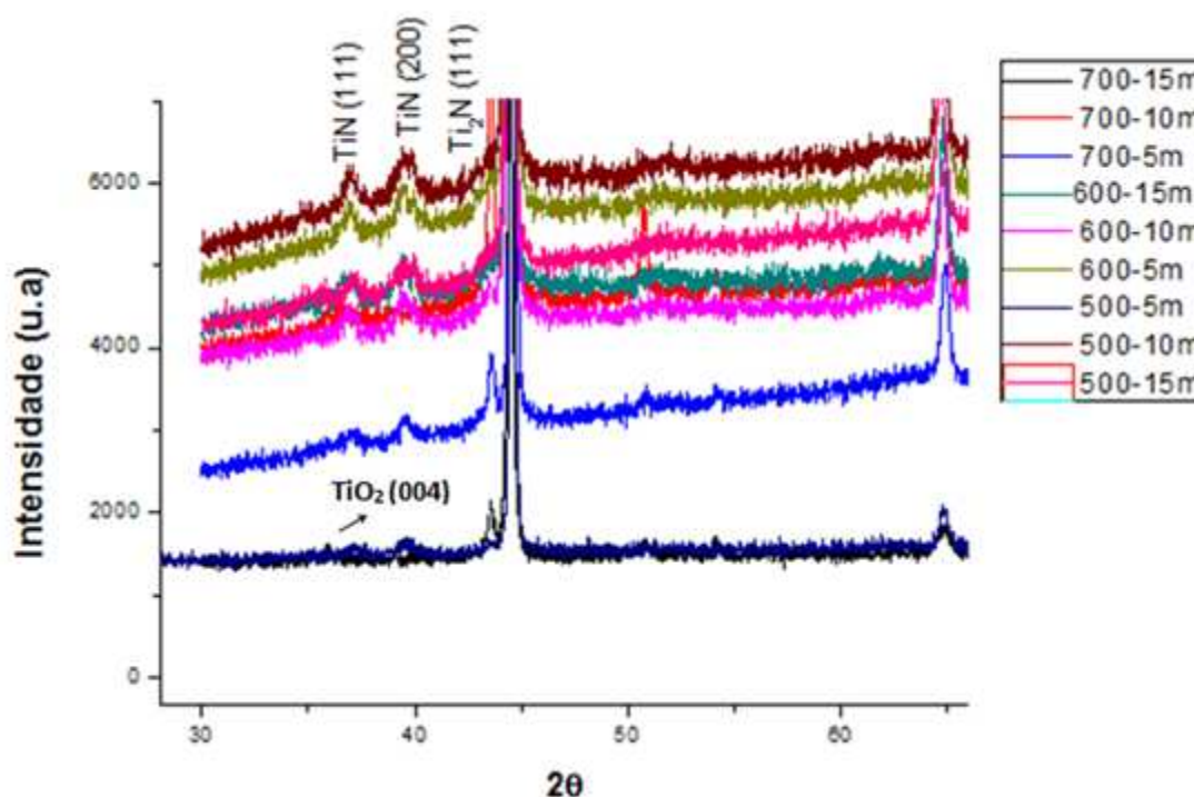
Figura 4.10: Difrátograma de raios X para as amostras tratadas em diferentes temperaturas e tempos, em atmosfera de nitrogênio.
