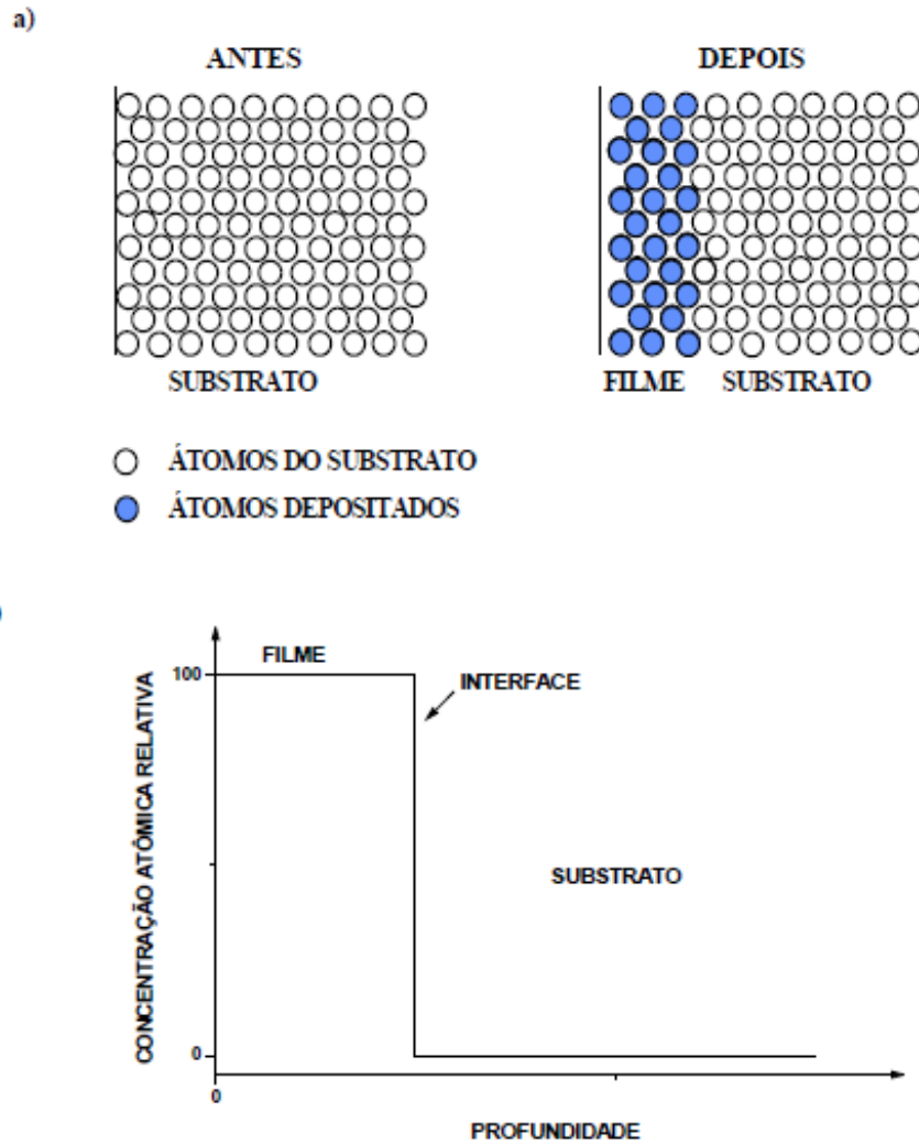
Figura 2.5: a) Distribuição característica dos átomos do filme e do substrato em técnicas com formação de interface definida e b) Representação gráfica da variação da concentração dos átomos do filme e do substrato em técnicas com formação de interface definida.
