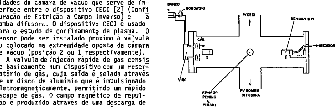
Fig. 1 - Esquema do sistema de medição da pressão de gás
