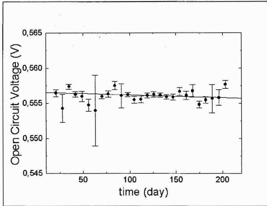
Figura 15 – Variação da tensão circuito aberto do ECS2 em função do tempo de vida do SCD2.
