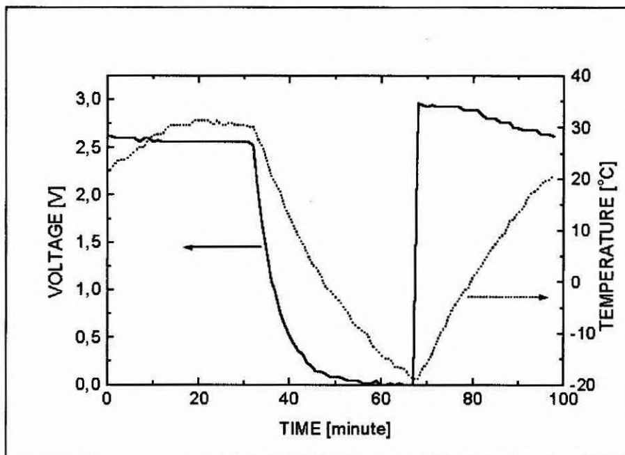
Figura 5 - Sinal e temperatura do ECS1 em função do tempo de órbita.
