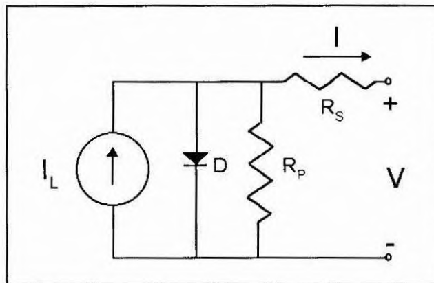
Figura 1 – Circuito elétrico equivalente de uma célula solar.
