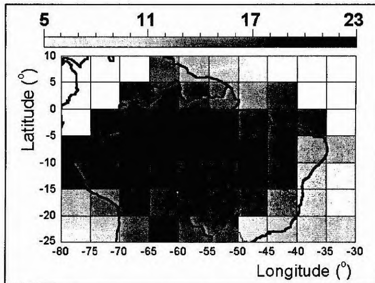
Figura 20 – Imagem do albedo planetário, valores mínimos, para o período do verão de 1999.
