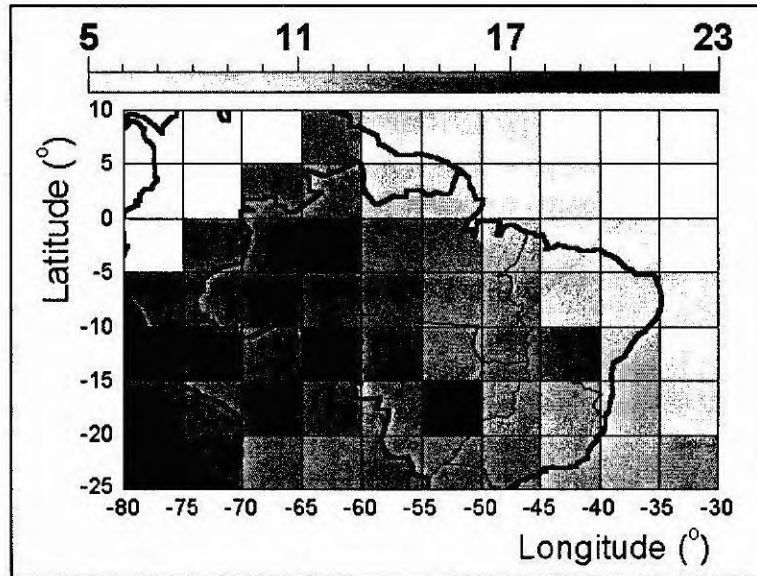
Figura 19 – Imagem do albedo planetário, valores mínimos, para o período da primavera de 1998.
