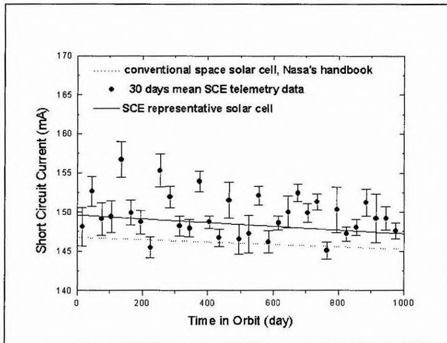
Figura 10 - Variação da corrente de curto circuito do ECS1 em função do tempo de vida do SCD1.
