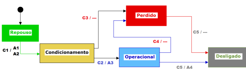
Figura 18: Estados de operação. (C=condição / A=Ação – Encontra-se na Tabela 1)
