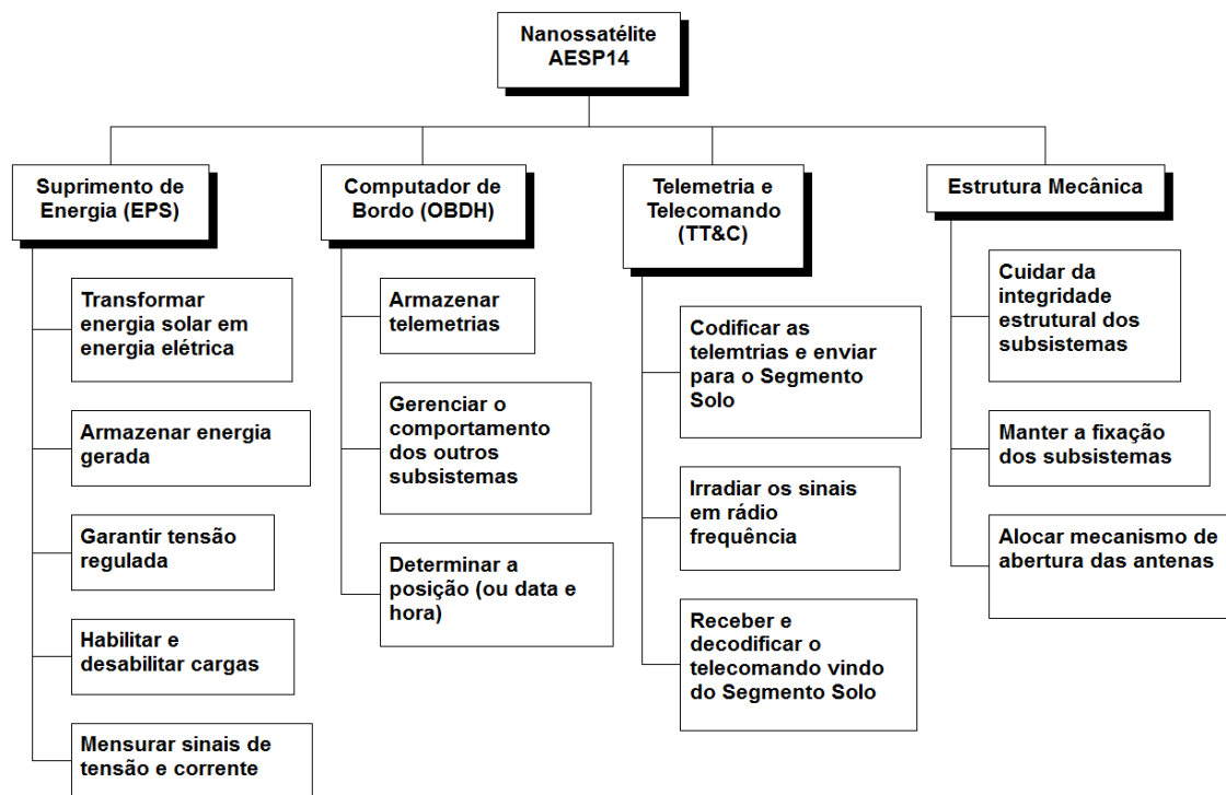
Figura 29. Alocação funcional a cada subsistema do satélite.
