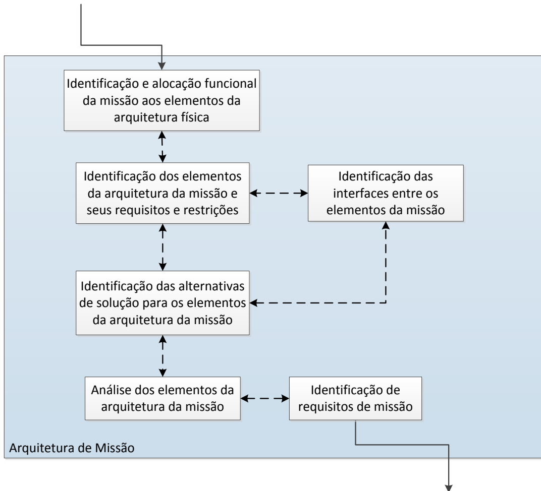
Figura 5.12 - Fluxograma das iterações das micro atividades da arquitetura de missão.
