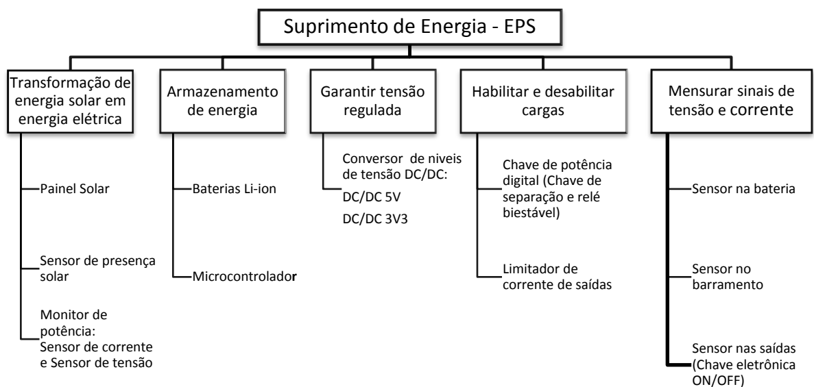
Figura 40 – Estrutura de alocação funcional do subsistema de suprimento de energia.
