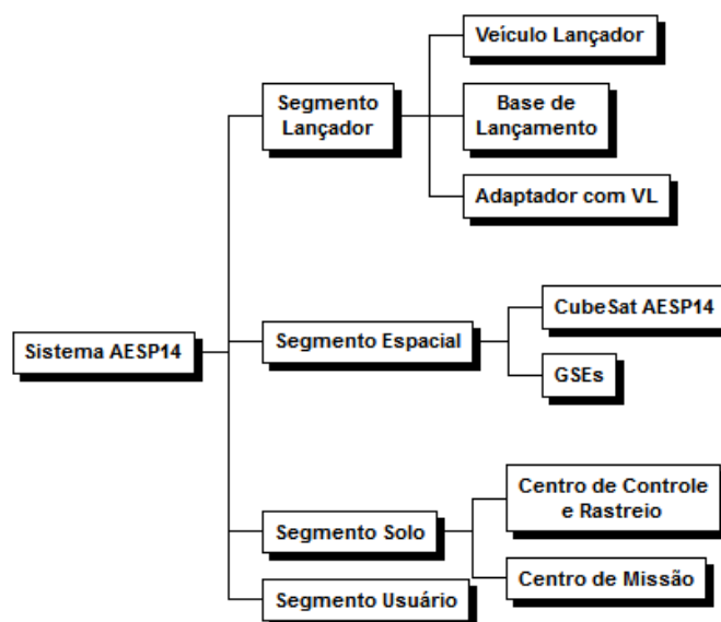
Figura 42: Arquitetura física da Missão AESP14
