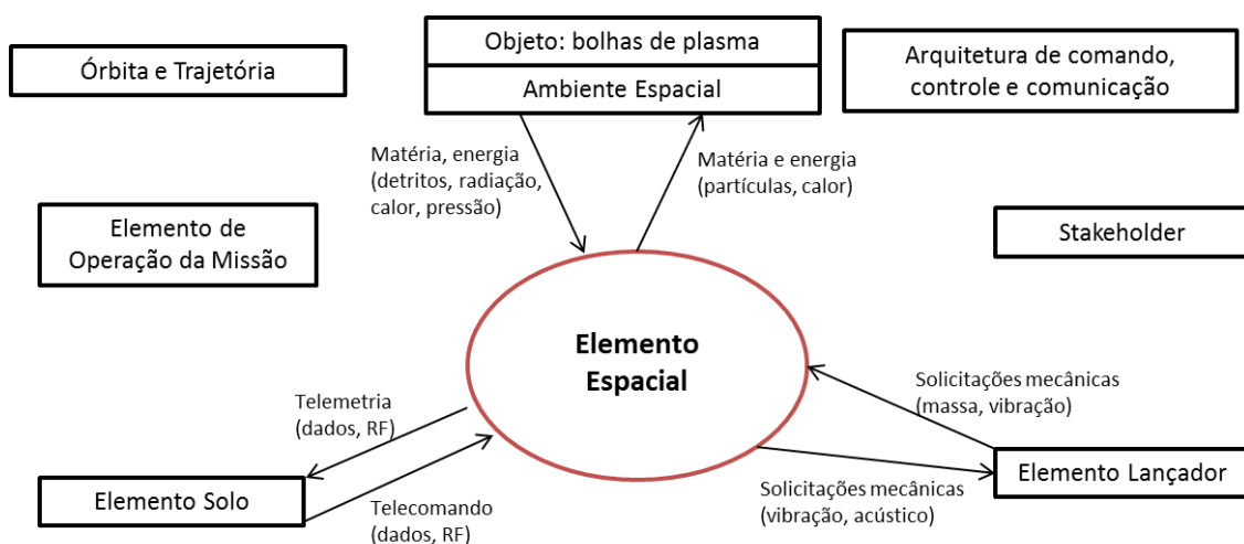
Figura 5.16 – Exemplo de diagrama de contexto para identificação de interfaces do elemento espacial.
