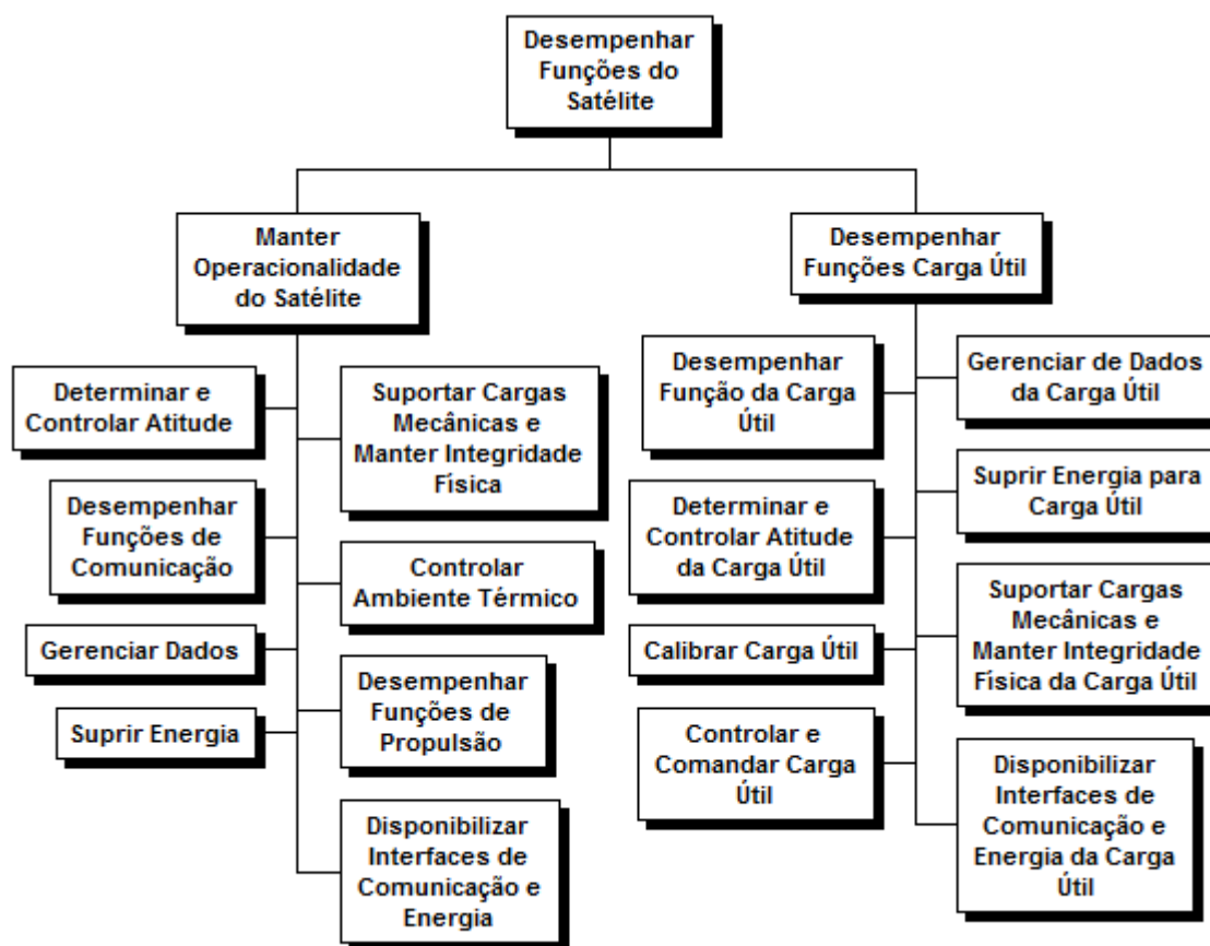
Figura 5.41 – Exemplo de arquitetura funcional genérica de um pico ou nano-satélite.
