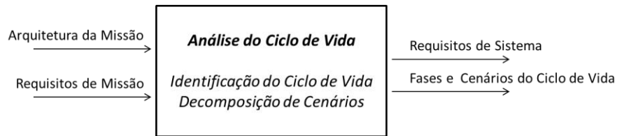
Figura 49. Processo de análise do ciclo de vida.
