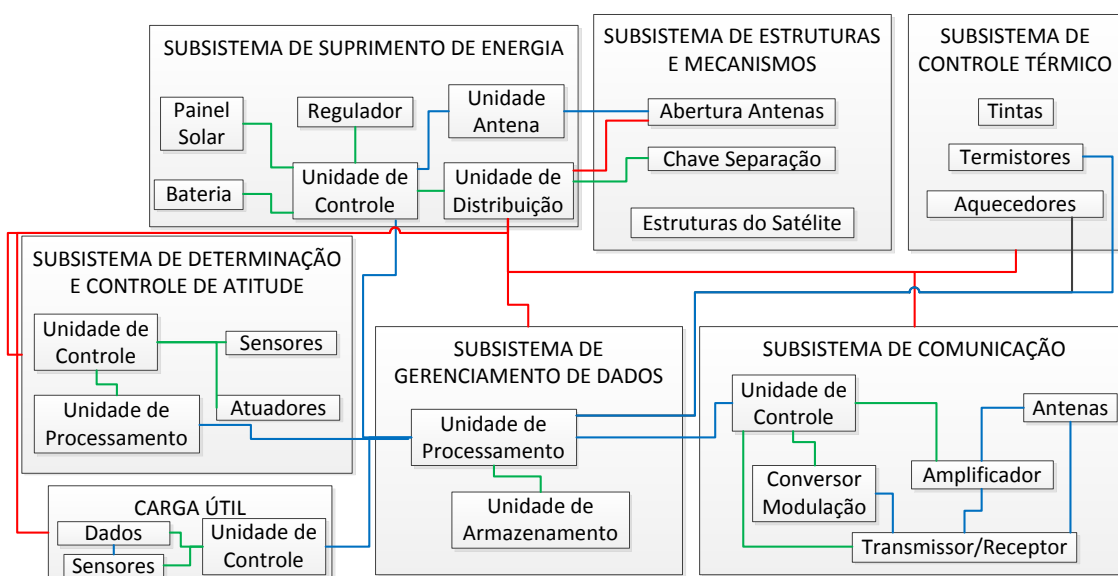
Figura 5.45 - Exemplo de diagrama de blocos do sistema CubeSat.
