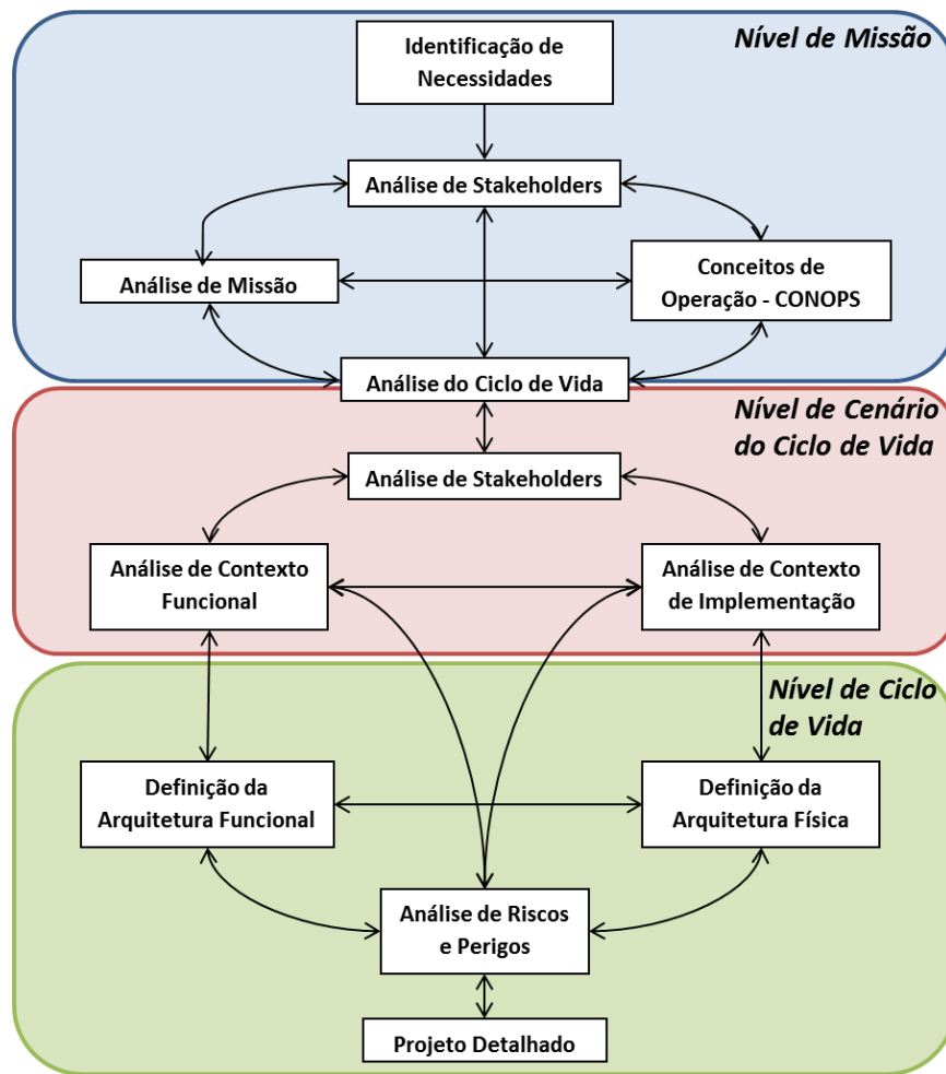
Figura 45. Processo de engenharia de sistemas adotado para o Projeto AESP14.
