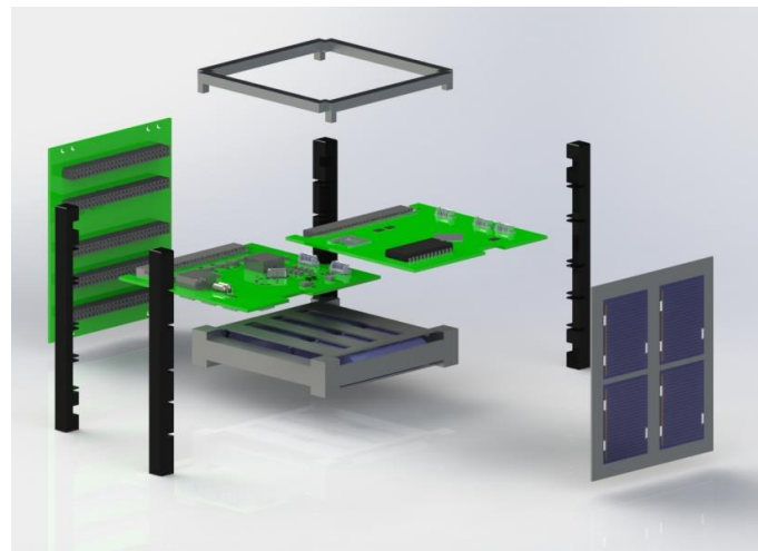
Figura 24: Diagrama explodido do satélite AESP14
