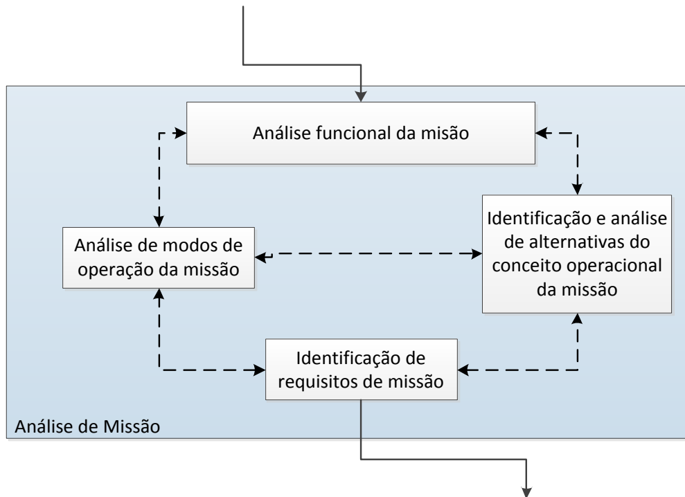
Figura 5.7 - Fluxograma de relacionamento das microatividades da análise de missão.
