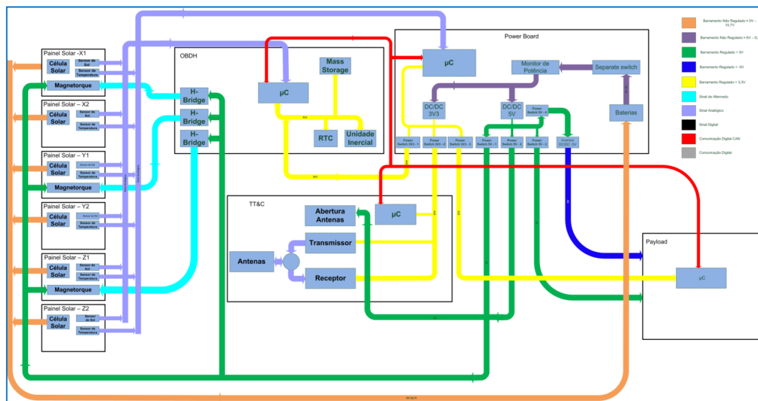
Figura 22: Arquitetura do CubeSat AESP14.
