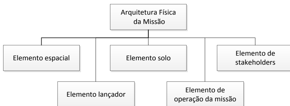
Figura 5.13 - Exemplo de arquitetura física de uma missão espacial.
