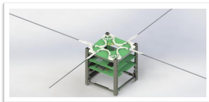
Figura 38 – Dispositivo de ejeção de antenas.
