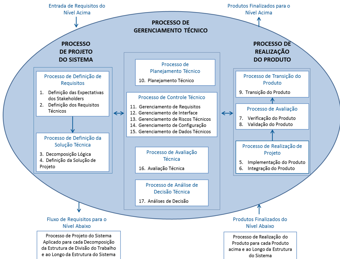
Figura 2.6 - Processo de engenharia de sistemas adotado pela NASA.
