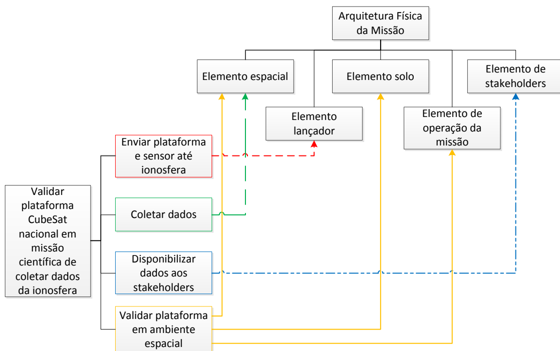
Figura 5.14 – Exemplo de alocação funcional para uma missão CubeSat.
