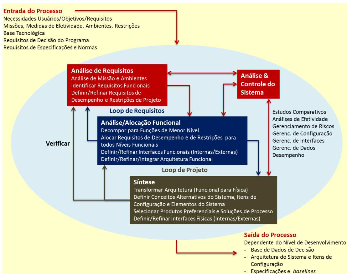
Figura 2.4 - Processo de engenharia de sistemas da SMC.
