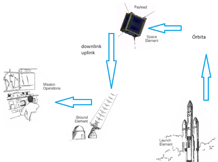
Figura 4: Arquitetura Operacional da Missão AESP14
