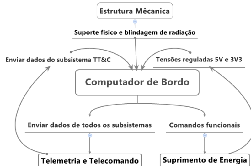
Figura 27 – Diagrama de interface do subsistema OBDH.
