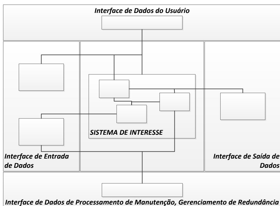
Figura 5.44 – Modelo de diagrama de interconexão de arquitetura – DIA.
