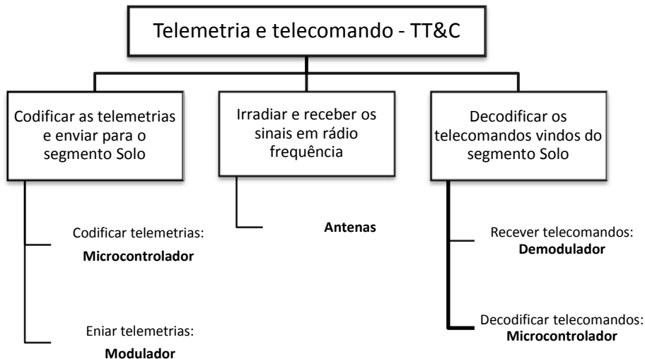
Figura 31. Alocação funcional aos elementos físicos do subsistema de telemetria e telecomando.
