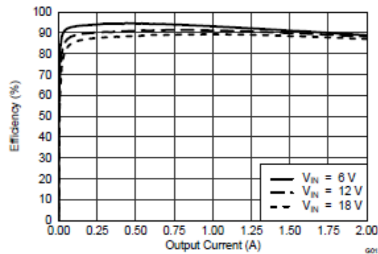
Figura 41 – Eficiência do conversor DC/DC utilizado no EPS.
