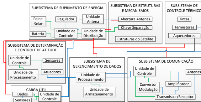
Figura B.7 – Modelo de apresentação da arquitetura de um satélite.
