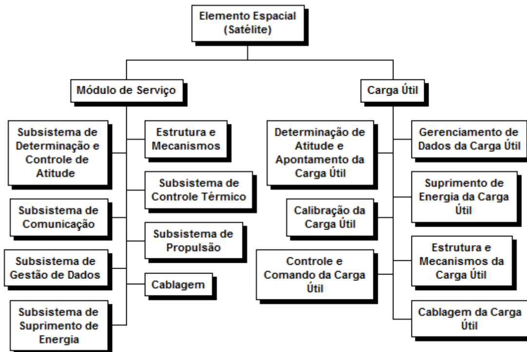
Figura 5.40 – Exemplo de arquitetura física genérica de um pico ou nano-satélite.
