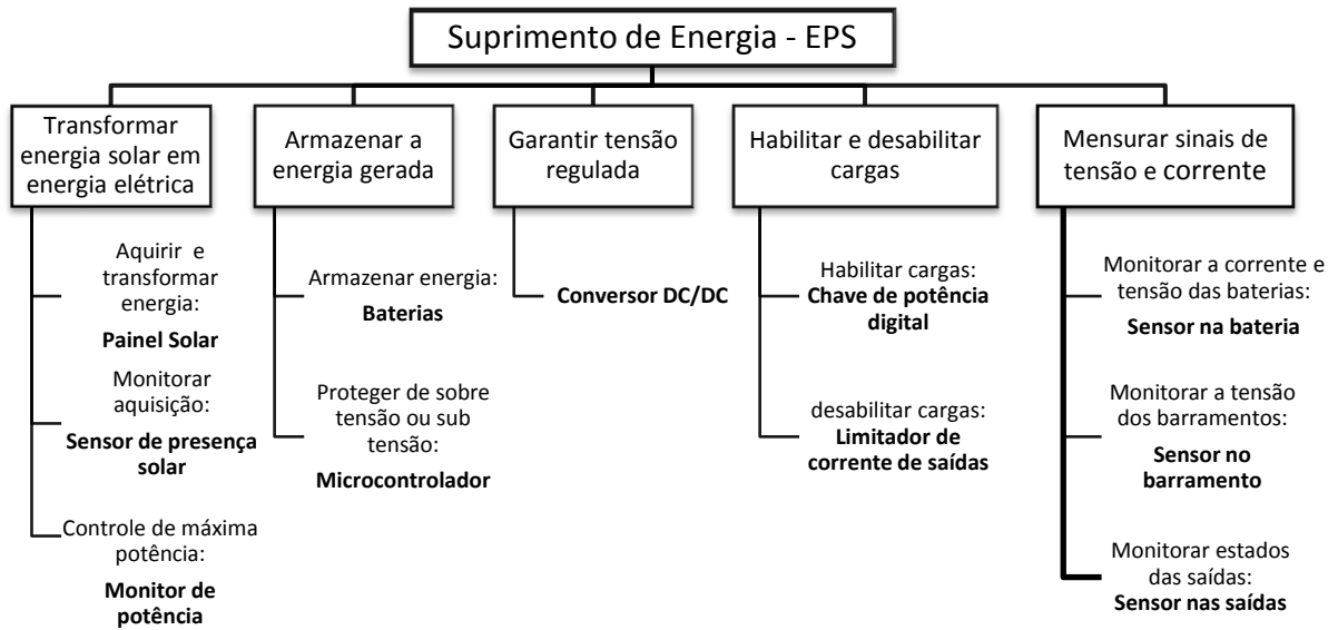
Figura 30. Alocação funcional aos componentes do subsistema de suprimento de energia.
