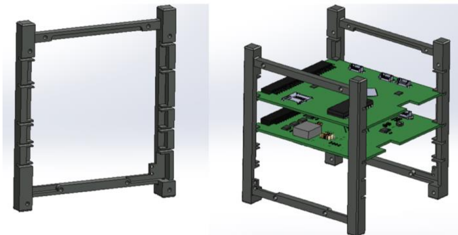
Figura 35 – Trilhos e o encaixe das PCBs.
