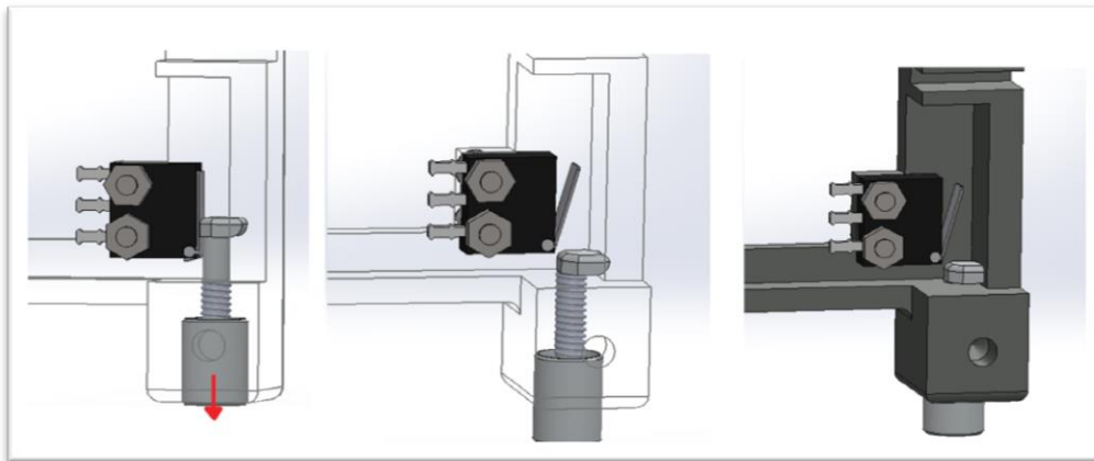
Figura 37 – Funcionamento do mecanismo Kill Switch .
