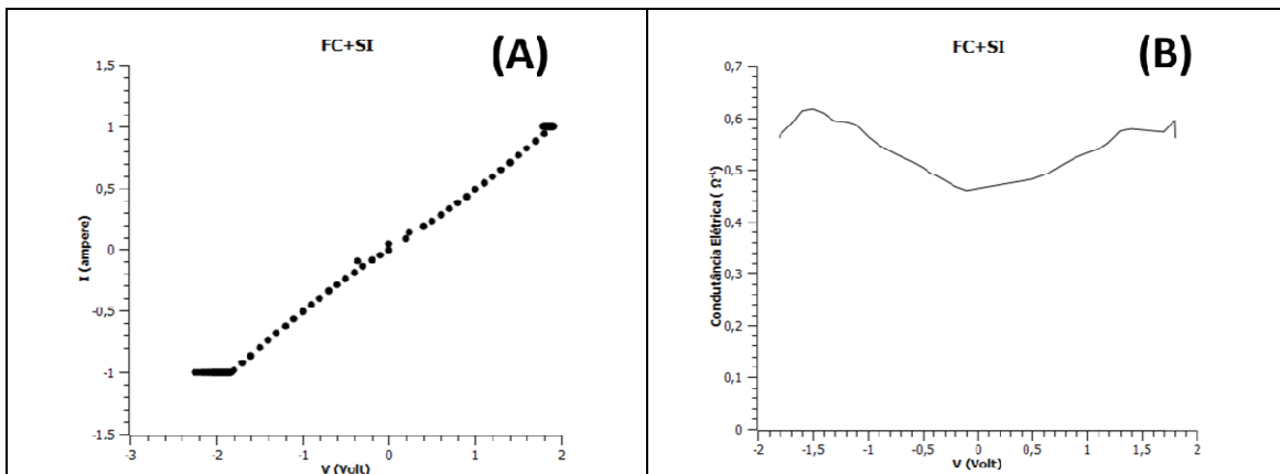
Figura 4.18: (A) Gráfico de corrente em função do potencial, medido no sentido horizontal, da amostra FC+Si - Fibra de carbono revestida com Si e resina (B) Gráfico da diferencial de corrente em função do potencial, medido no sentido horizontal, da amostra FC+Si - fibra de carbono revestida com Si e resina.
