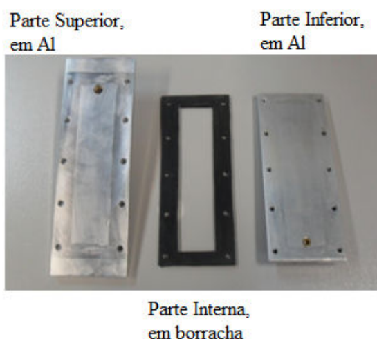
Figura 3.7: Foto das partes separadas do molde confeccionado
