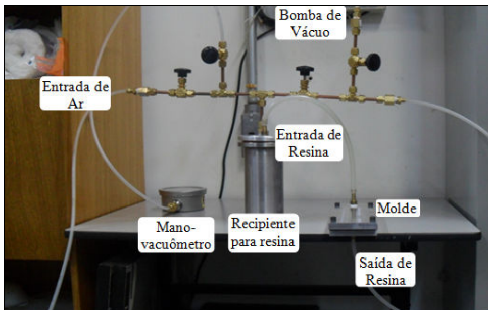
Figura 3.6: Foto do molde para confecção dos compósitos
