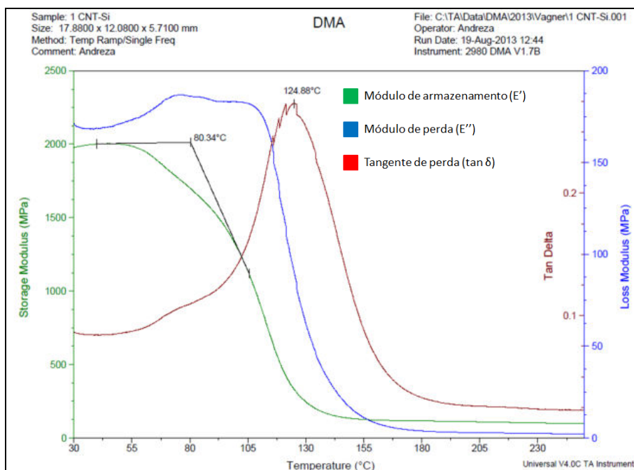
Figura 4.15 - Curvas obtidas pela técnica de DMA do compósito: (D) FC+Si+CNT+Si (Si amorfo depositado sobre CNT crescido sobre a FC revestida com Si amorfo e resina)
