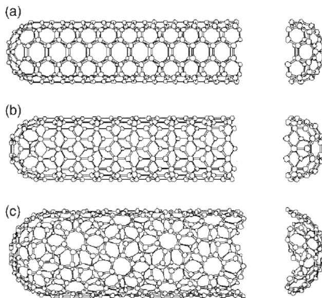
Figura 2.4: Estruturas geométricas de SWCNT. (a) CNT armchair (5,5), (b) CNT zigzag (9,0) e (c) CNT chiral (10,5).
