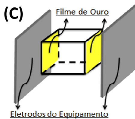
Figura 3.13: Imagens ilustrativas das características das medidas elétricas. (A) Dimensões da amostra, (B) Deposição do filme de ouro, (C) Detalhe dos eletrodos do equipamento.
