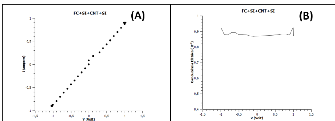
Figura 4.20: (A) Gráfico de corrente em função do potencial, medido no sentido horizontal, da amostra FC+Si+CNT+Si - Si amorfo depositado sobre CNT crescido sobre a FC revestida com Si e resina (B) Gráfico da diferencial de corrente em função do potencial, medido no sentido horizontal, da amostra FC+Si+CNT+Si - Si amorfo depositado sobre CNT crescido sobre a FC revestida com Si amorfo e resina.
