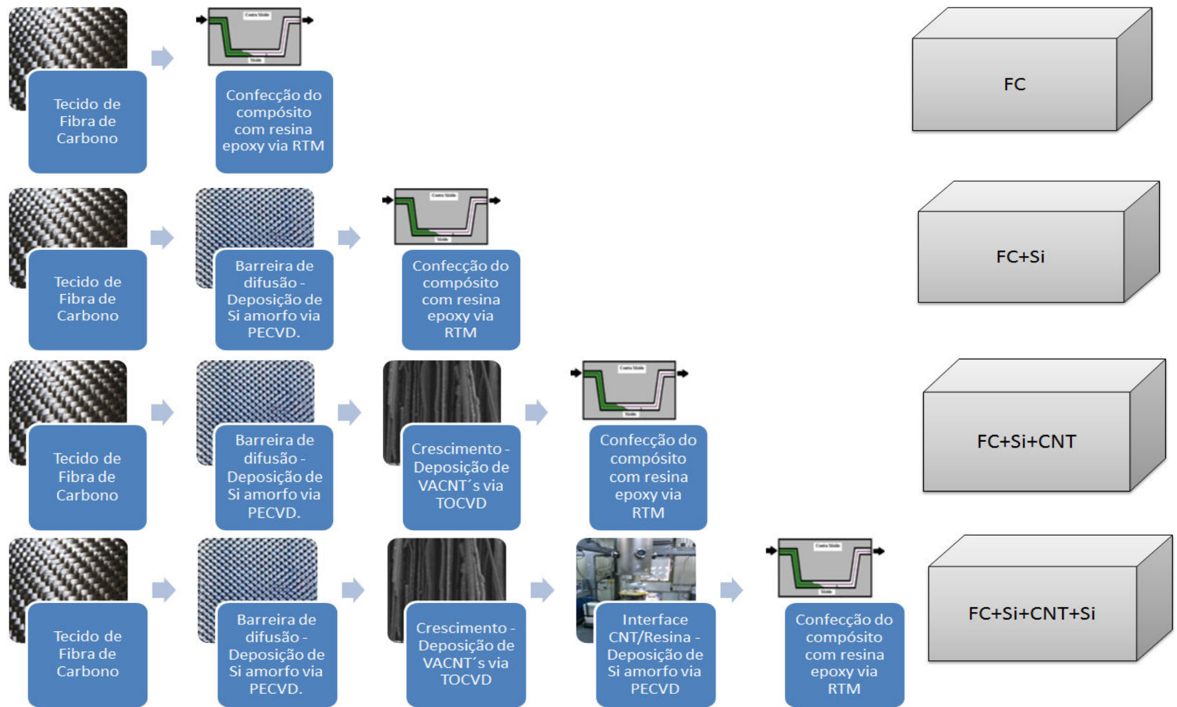
Figura 3.9: Fluxograma de obtenção dos diversos tipos de amostras.
