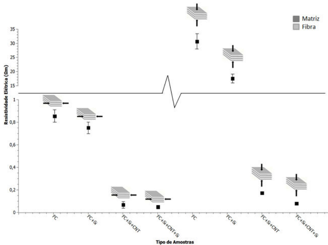
Figura 4.26: Imagem da resistividade elétrica das amostras medidas no sentido horizontal e vertical as fibras de carbono.
