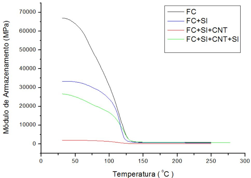
Figura 4.16 – Curvas obtidas pela técnica de DMA do Módulo de armazenamento das amostras FC, FC+Si, FC+Si+Si e FC+Si+Si+Si obtidos das curvas da Figura 4.14.
