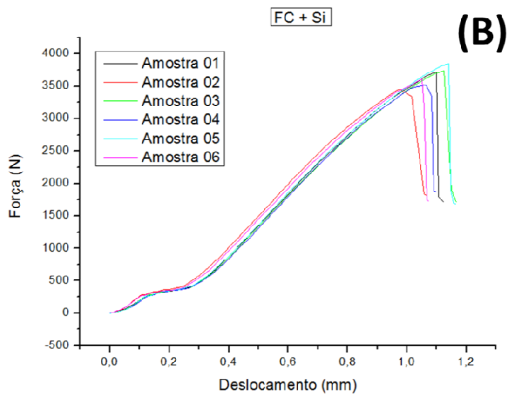
Figura 4.13: Curvas obtidas pela técnica de Cisalhamento Interlaminar das amostras (B) FC+Si (Fibra de carbono revestida com Si e resina)
