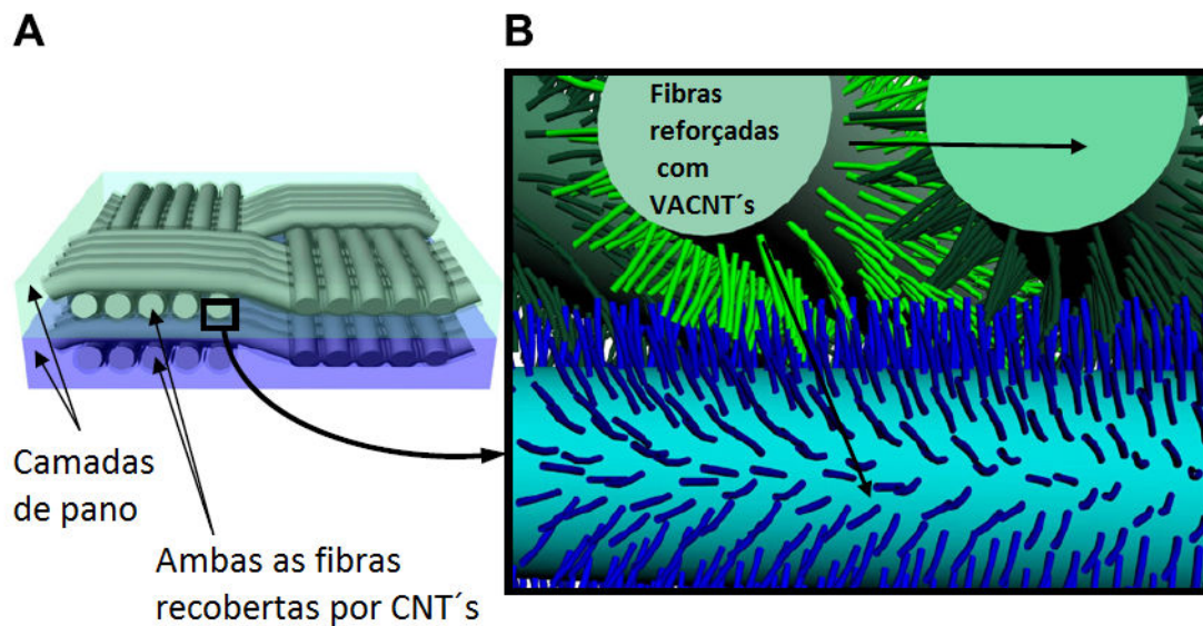
Figura 2.8 – Ilustração esquemática da FuzzyFiber. (A) Arquitetura de um compósito de fibras de carbono revestidas com VACNT's em uma matriz polimérica. (B) Visão aproximada das camadas internas do compósito contendo os VACNT's crescidos sobre as fibras. Adaptado de
