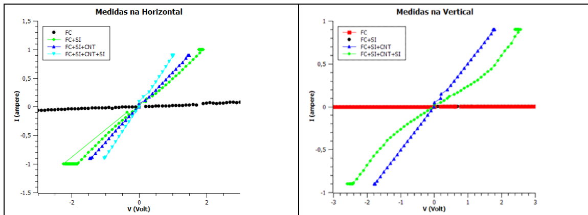
Figura 4.25: Gráfico de corrente em função do potencial, medido no sentido paralelo (A) e perpendicular (B), das amostras FC, FC+SI, FC+SI+CNT e FC+SI+CNT+SI.
