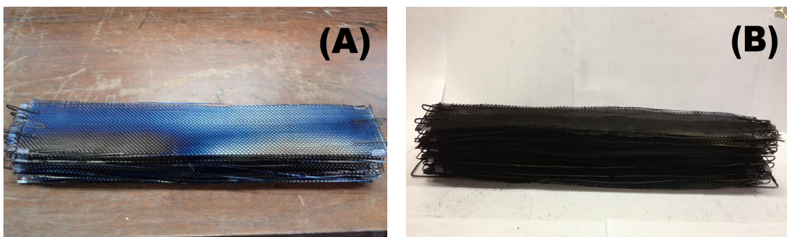
Figura 4.3: Foto do detalhe da disposição das fibras sobre o dispositivo utilizado para escalonamento do processo, fibras de carbono antes (A) e depois (B) do crescimento de CNT no TOCVD.
