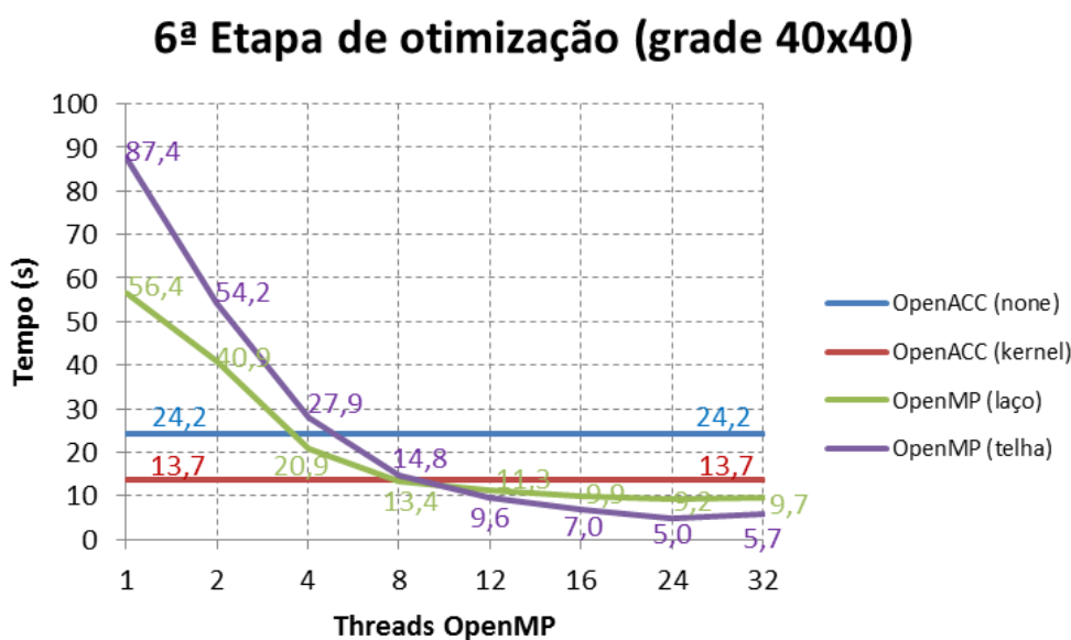
Figura 5.15 – Comparação dos tempos de execução das versões OpenMP por laços e por telhas 2x2 em função do número de threads com o tempo de execução das versões da 6ª etapa do OpenACC com opções de compilação async_kernel e async_none .
