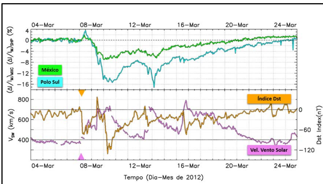
Figura 6.2 – Comparação entre a variação em relação à média dos dias anteriores da intensidade de raios cósmicos observada pelo monitores de nêutrons localizados no México (\Delta I/I)_{MEX} e no Polo Sul (\Delta I/I)_{SPH} durante o Decréscimo de Forbush ocorrido no dia 08 de março de 2012. No quadro superior, a linha verde representa os dados observados no México, enquanto a linha ciano representa os dados coletados no Polo Sul. No quadro inferior, a linha laranja representa os valores do Índice Dst, a linha lilás representa o módulo da velocidade do vento solar ( V_{SW} ), os triângulos laranja e violeta indicam respectivamente o registro de um início súbito de tempestade (SSC) e de um choque interplanetário.
