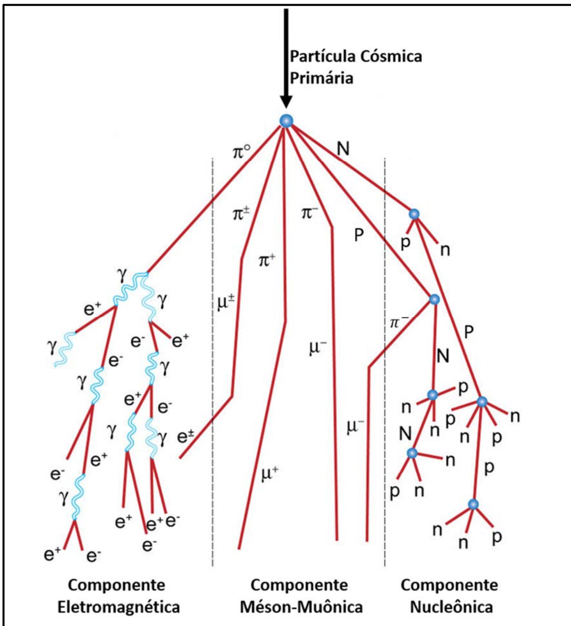
Figura 1.14 – Esquema do Chuveiro de Raios Cósmicos produzido por uma partícula primária, ao entrar na atmosfera terrestre, onde: “n” são nêutrons, “p” são prótons, “e-” são elétrons, “e+” são pósitrons, “π” são píons, “μ” são múons, “γ” são fótons, “N” e “P” representam nêutrons e prótons de alta energia. Fonte: Modificado de Otaola & Valdés-Galicia (1995).
