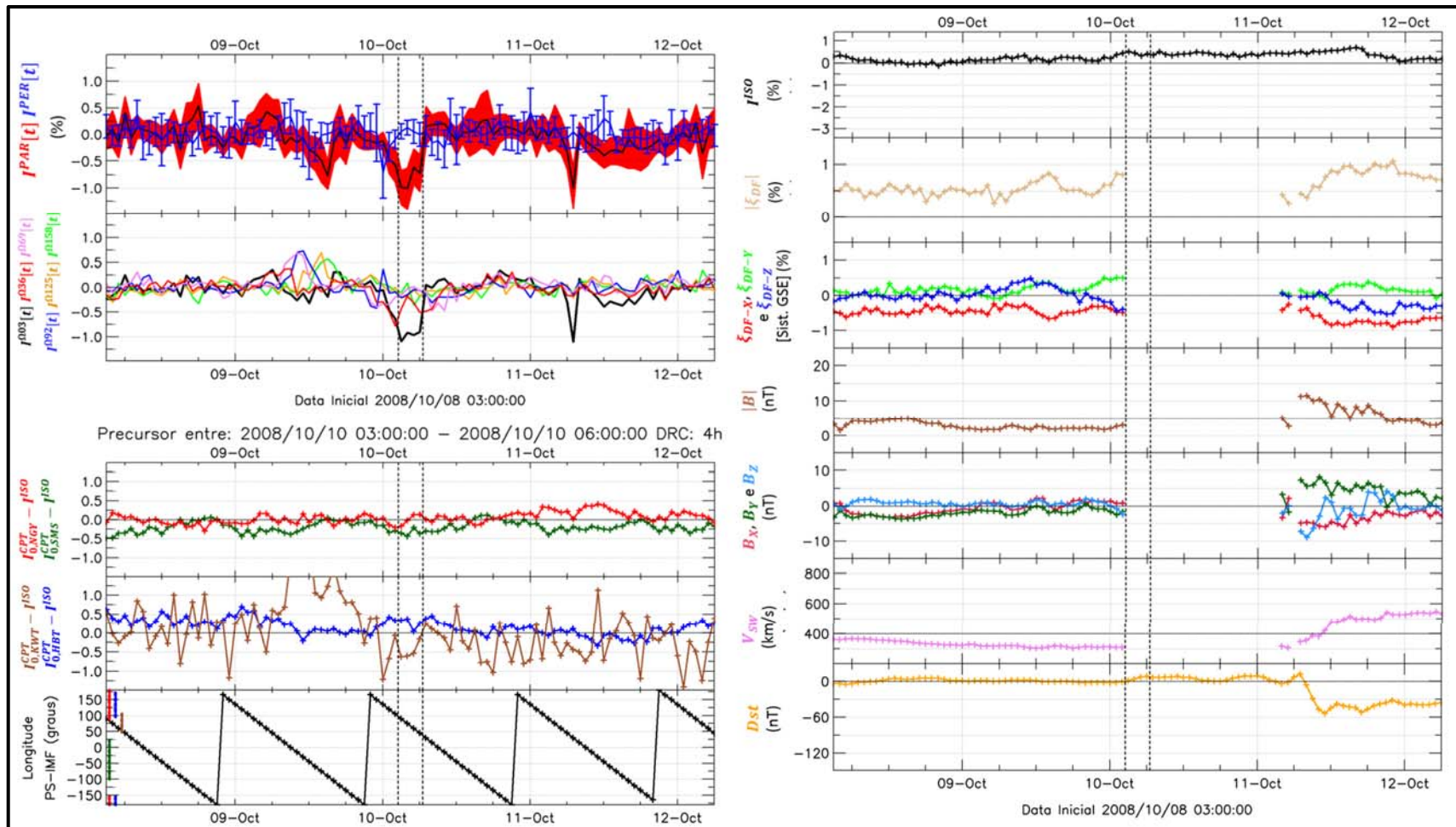
Figura 6.22 – Exemplo da seleção automática de um provável decréscimo precursor num período onde não há dados do módulo e das três componentes do campo magnético interplanetário ( |\vec{B}| , B_x , B_y e B_z ) e da velocidade do vento solar ( |\vec{V}_{sw}| ), que dizem respeito à situação do meio interplanetário neste período.
