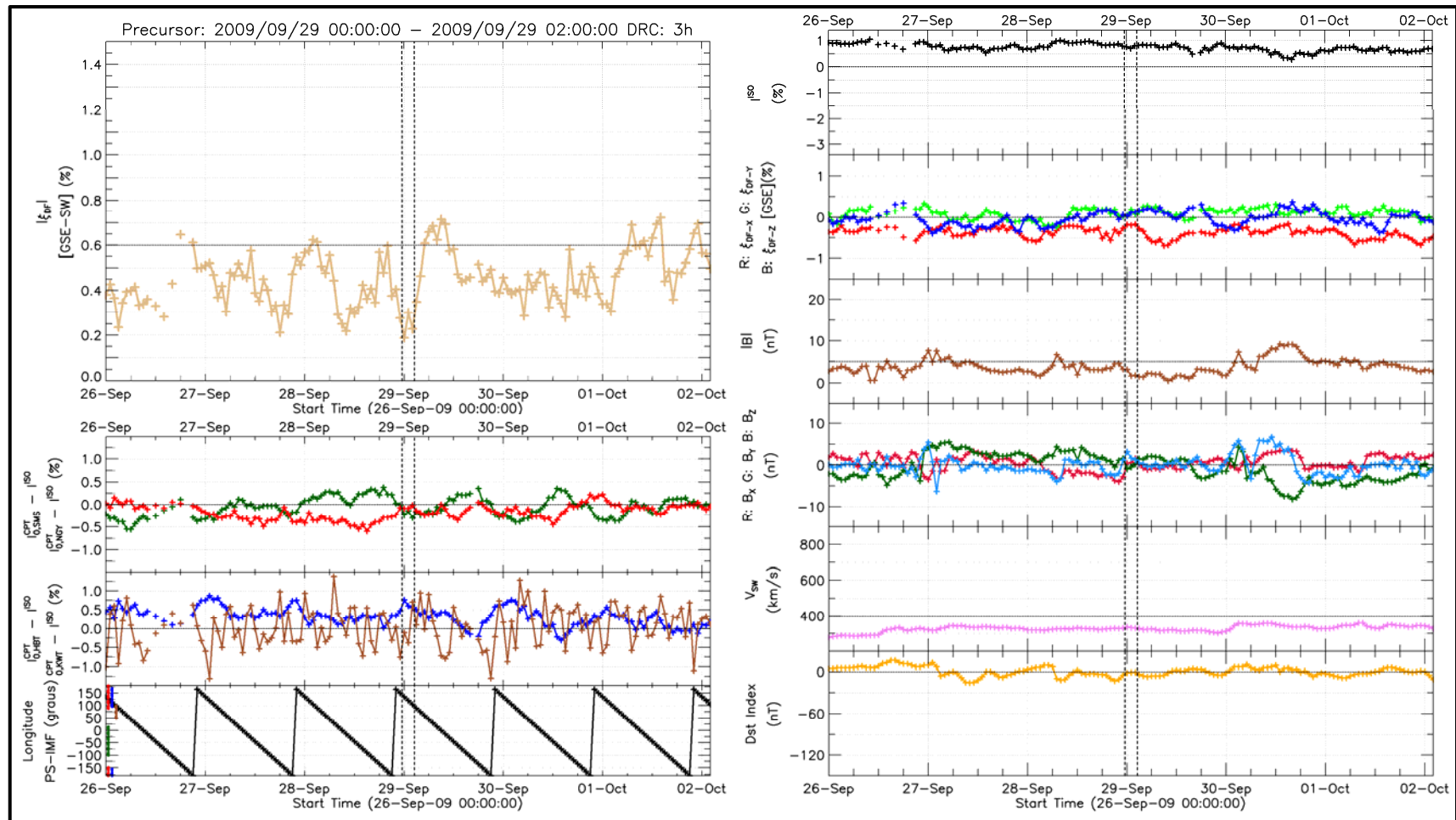
Figura 6.36 – Exemplo da seleção automática de um provável acréscimo precursor num período onde o módulo do vetor anisotropia devido a difusão ( |\xi_{DF}^2| ) parece estar oscilando, e não diminuindo (como se espera que ocorra durante um acréscimo precursor).
