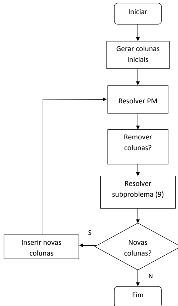
Figura 1: Algoritmo GC.
