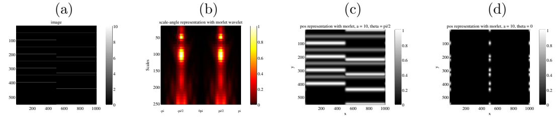
Figura 3: Imagem com várias linhas(a). Média da representação de escala-ângulo da CWT com wavelet de Morlet (b). CWT em representação de posição, com \theta = \pi/2 e \theta = 0 respectivamente (c, d).
