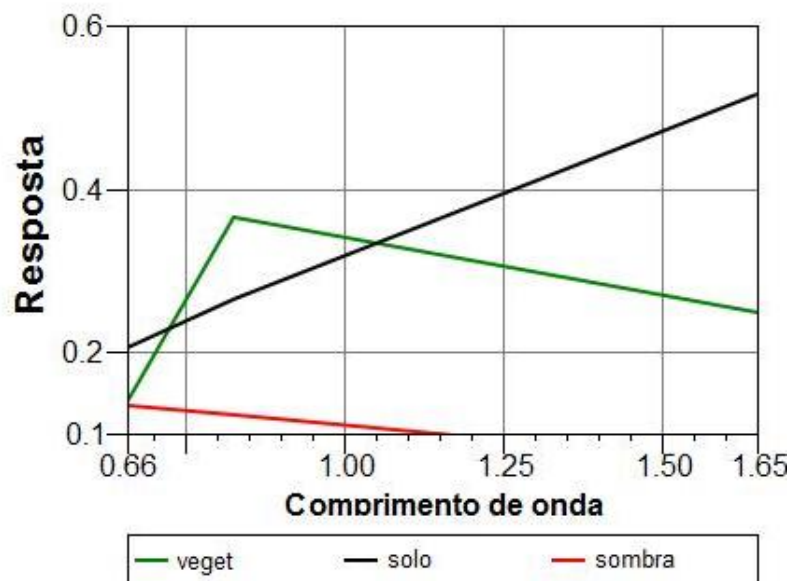
Figura 4.3 – Curva de reflectância dos pixels puros de referência (Espectro derivado da cena TM/Landsat de código LT52270652005198CUB00, ver Tabela 4.2)
