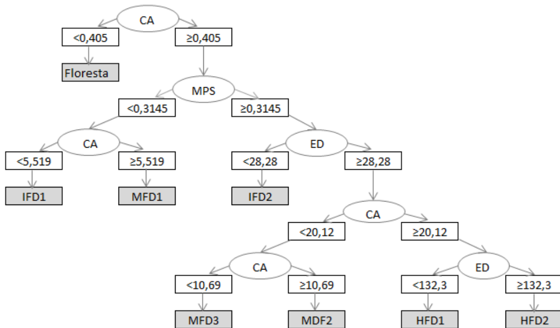
Figura 5.1 - Árvore de decisão para a classificação de padrões espaciais de degradação florestal em Novo Progresso, PA. (As métricas de paisagem são: CA, área da classe (ha); ED, densidade de borda (m/ha); MPS, tamanho médio das manchas (ha). Os padrões espaciais classificados são: LFD1: degradação florestal de intensidade baixa–1; LFD2: degradação florestal de intensidade baixa–2; MFD1: degradação florestal de intensidade moderada–1; MFD2: degradação florestal de intensidade moderada–2; MFD3: degradação florestal de intensidade moderada–3; HDF1: degradação florestal de intensidade alta–1; HDF2: degradação florestal de intensidade alta–2)
