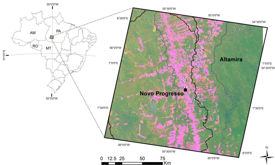
Figura 3.2 – Localização da área de estudo (Órbita/Ponto 227/65 do sensor TM/Landsat, ano 2011) no estado do Pará: Novo Progresso e região
