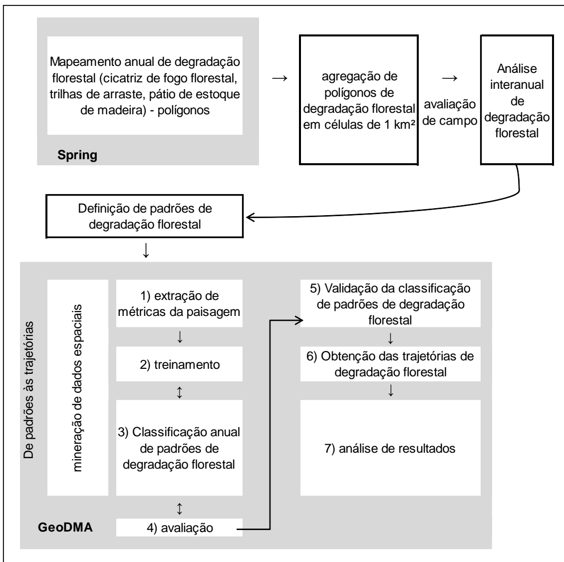
Figura 4.1 – Fluxograma descritivo das principais etapas metodológicas do estudo
