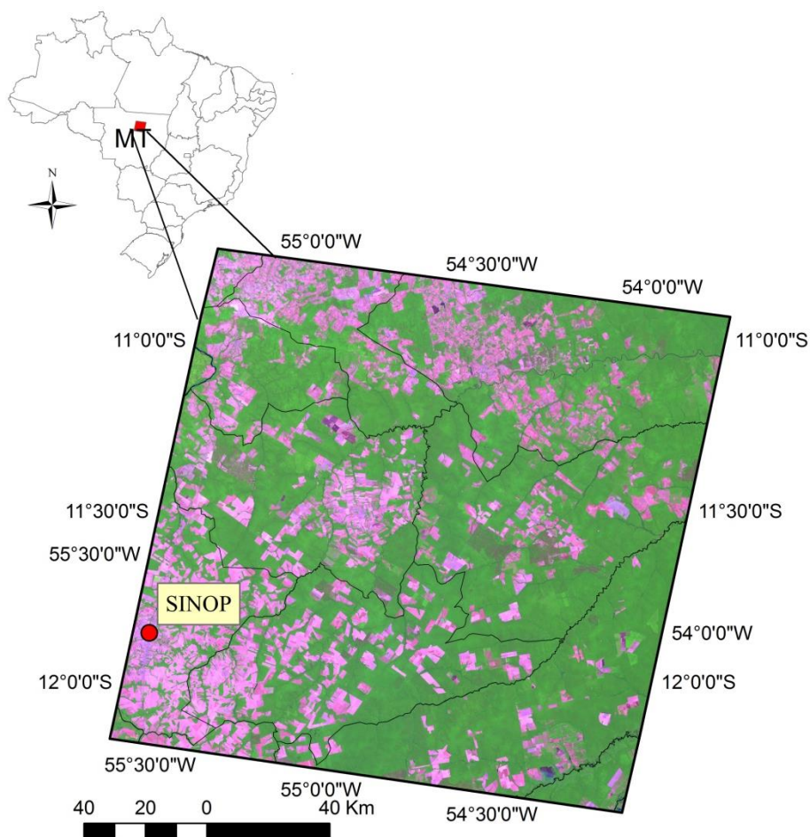
Figura 3.1 – Localização da área de estudo (Órbita/Ponto 226/68 do sensor TM/Landsat, ano 2011) no estado do Mato Grosso: Sinop e região (MT)
