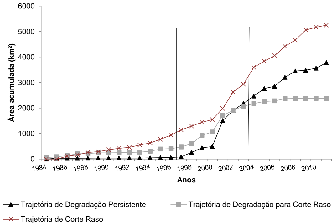
Figura 5.4 – Trajetórias de mudança de cobertura da terra: Evolução anual entre 1984 e 2011, em Novo Progresso (PA) (barras verticais marcam três períodos: 1984 a 1997; 1998 a 2004; 2005 a 2011)
