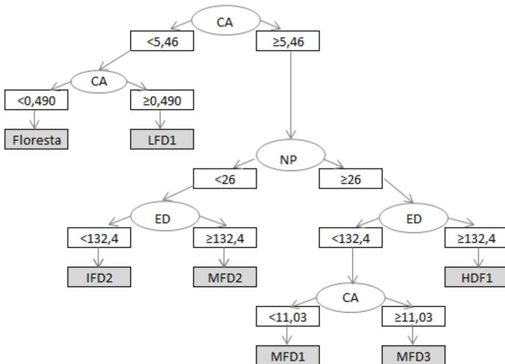
Figura 5.12 - Árvore de decisão para classificação de padrões espaciais de degradação florestal em Sinop, Mato Grosso. (As métricas de paisagem são: CA, área da classe (ha); ED, densidade de borda (m/ha); NP, número de manchas (NP \geq 1, sem limite). Os padrões espaciais são: LFD1: degradação florestal de intensidade baixa-1; LFD2: degradação florestal de intensidade baixa-2; MFD1: degradação florestal de intensidade moderada-1; MFD2: degradação florestal de intensidade moderada-2; MFD3: degradação florestal de intensidade moderada-3; HDF1: degradação florestal de intensidade alta-1; HDF2: degradação florestal de intensidade alta-2)
