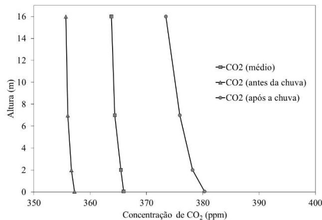
Figura 3. Perfil da concentração de dióxido de carbono ( \text{CO}_2 , ppm) em uma área de caatinga preservada, Petrolina, PE.
