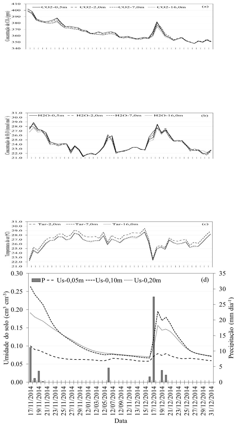
Figura 1. Média diária da concentração de dióxido de carbono (CO 2 , ppm) (a); de vapor d'água (H 2 O, mmol mol -1 ) (b); temperatura do ar (Tar, °C) (c); da umidade do solo (Us, cm 3 cm -3 ) e total diário da precipitação (P, mm dia -1 ) (d), observados nas alturas de 0,5; 2,0; 7,0 e 16m acima da superfície do solo em uma área de caatinga preservada, Petrolina, PE.
