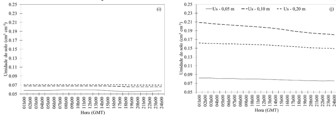
Figura 2. Concentração de dióxido de carbono ( \text{CO}_2 , ppm) (a e b); de vapor d'água ( \text{H}_2\text{O} , \text{mmol mol}^{-1} ) (c e d); temperatura do ar ( T_{\text{ar}} , ^{\circ}\text{C} ) (e e f); déficit de pressão de vapor d'água (kPa) (g e h) e umidade do solo ( U_s , \text{cm}^3 \text{cm}^{-3} ) (i e j), para os dias 15 (coluna da esquerda) e 18 (coluna da direita) de dezembro de 2014, observados nas alturas de 0,5; 2,0; 7,0 e 16m acima da superfície do solo em uma área de caatinga preservada, Petrolina, PE.
