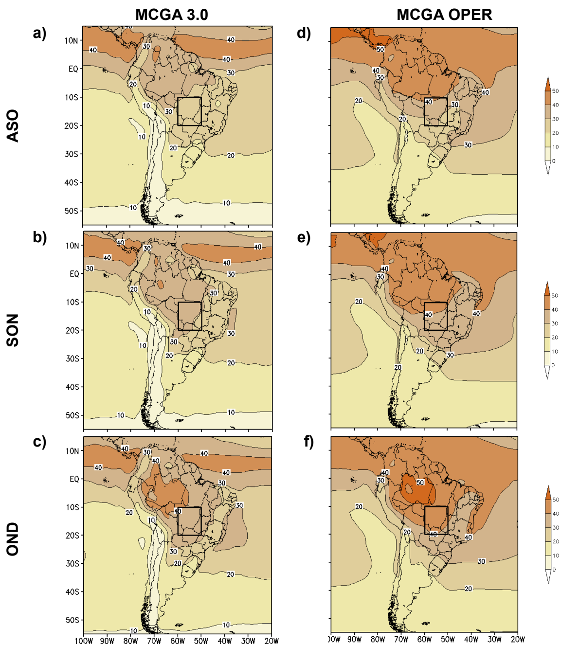
Figura 4.25 – Idem ao anterior, mas para a água precipitável ( \text{kg.m}^{-2} ).
