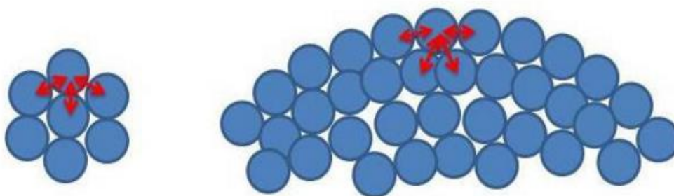
Figura 2.9 – Figura que ilustra o efeito de curvatura no número de ligações (flechas vermelhas) que uma molécula de água recebe. Maior curvatura implica em menos ligações com as moléculas vizinhas e a gota precisa de um ambiente com maior supersaturação para si manter.
