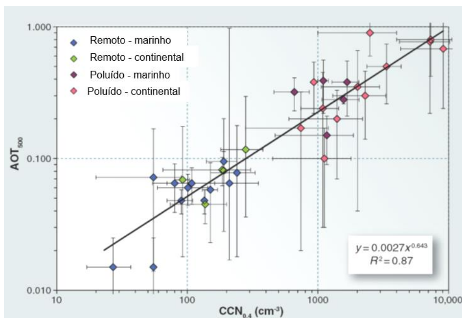
Figura 3.10 - Relação entre a POA em 500 nanômetros (Aerosol Optical Thickness, AOT) e da concentração numérica de CCNs ( CCN_{0,4} ) em cm^{-3} , obtidas sobre regiões remotas ou poluídas localizadas sobre continentes ou oceanos. As barras de erro representam a variação observada em medições realizadas por diversos estudos.
