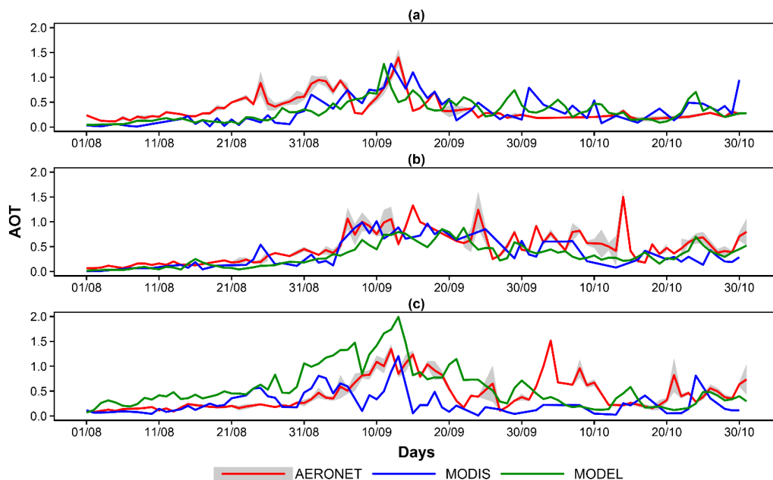
Figura 4.3 – Série temporal diária de POA para os sítios de Rio Branco (a), Cuiabá (b) e Alta Floresta (c) obtidas via AERONET, comparando seus resultados com os obtidos via MODIS e rodada MODEL CA para os pixels mais próximos dos sítios no período de agosto a outubro. O intervalo cinza nos dados da AERONET representa o desvio padrão da variação diária.
