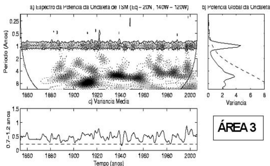
Figura 3 - Idem Figura 2, para a área 3 e \sigma^2 = 0,4525 .
