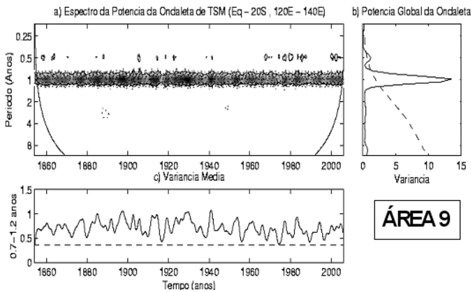
Figura 6 - Idem Figura 2, para a área 9 e \sigma^2 = 0,9160 .
