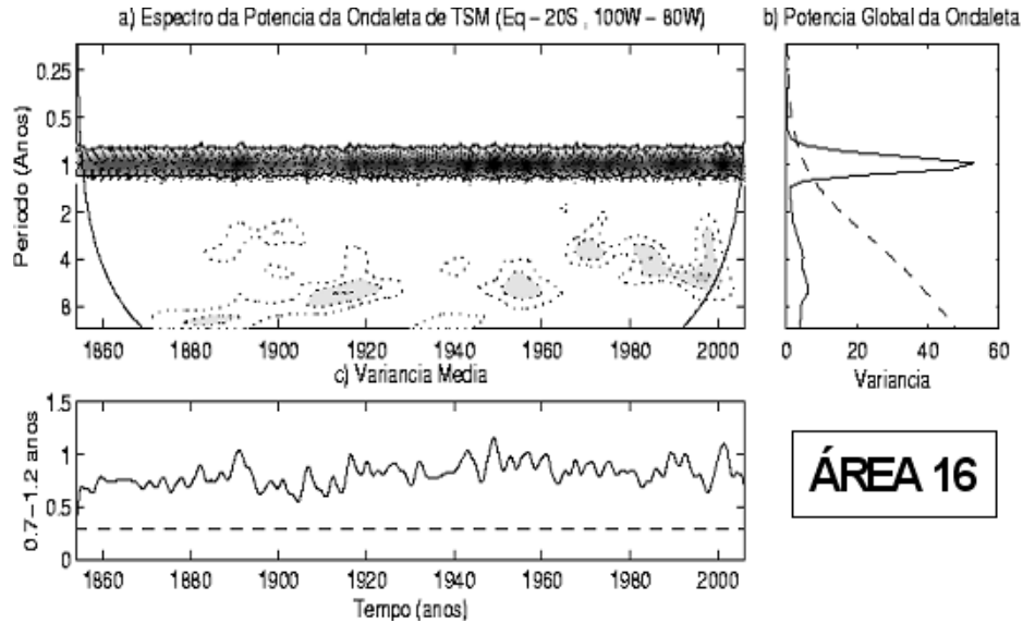
Figura 10 - Idem Figura 2, para a área 16 e \sigma^2 = 3,1444 .
