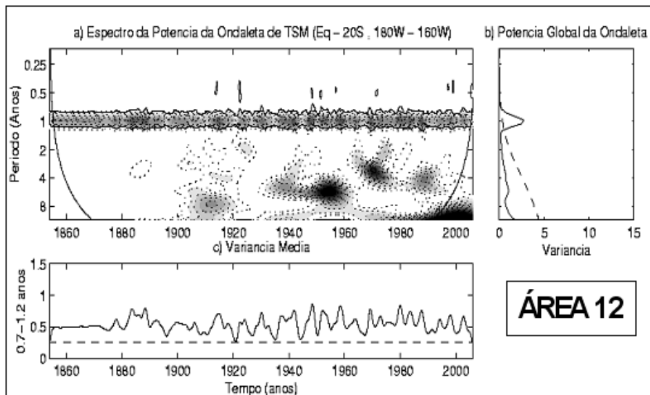
Figura 8 - Idem Figura 2, para a área 12 e \sigma^2 = 0,2463 .
