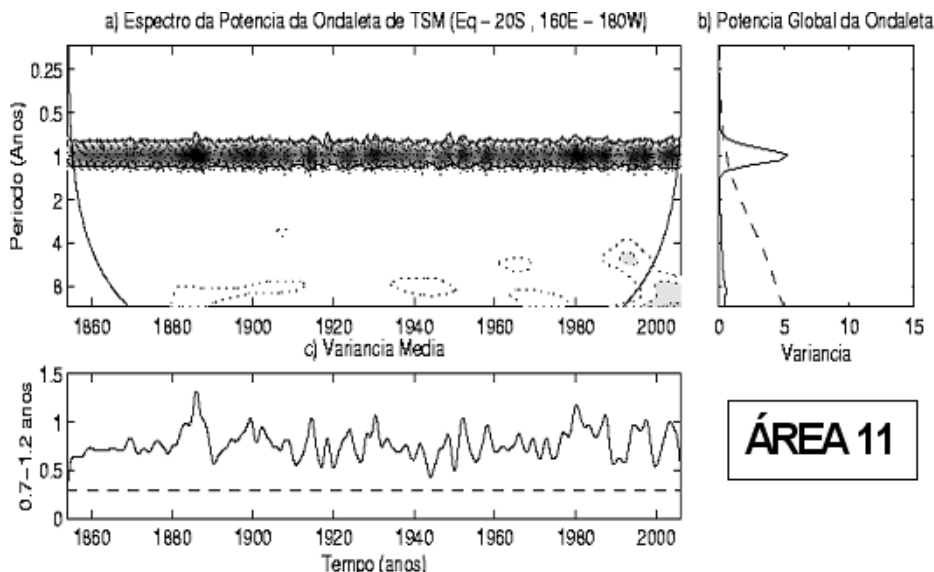
Figura 7 - Idem Figura 2, para a área 11 e \sigma^2 = 0,3304 .
