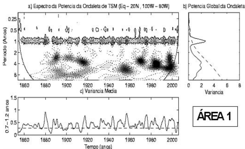
Figura 2 - a) EPO para o índice de TSM da área 1, normalizado por \sigma^2=0,3202 ; b) EPG; c) MEPO na banda de 0,7 – 1,2 anos. Em a) as áreas sombreadas representam variâncias normalizadas, variando de 0 a 20 com o intervalo de contorno de 2, a curva em forma de U representa o COI, e os contornos fechados indicam áreas com EPO significativo ao nível de confiança de 95%. Em (b), à direita da curva tracejada, o EPG é significativo ao nível de confiança de 95%. Em (c), acima da reta tracejada a MEPO é significativo ao nível de confiança de 95%.
