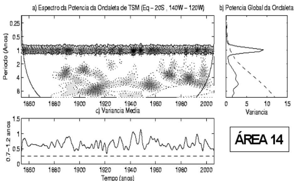
Figura 9 - Idem Figura 2, para a área 14 e \sigma^2 = 0,6796 .
