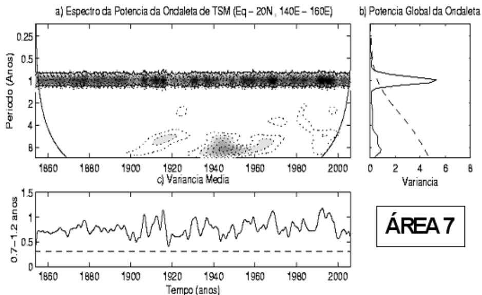
Figura 5 - Idem Figura 2, para a área 7 e \sigma^2 = 0,3339 .
