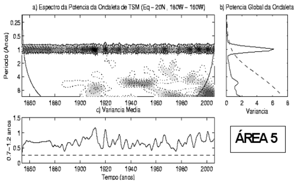
Figura 4 - Idem Figura 2, para a área 5 e \sigma^2 = 0,4351 .
