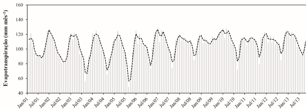
Figura 5.14 - Evapotranspiração mensal entre janeiro de 2001 e dezembro de 2013.
