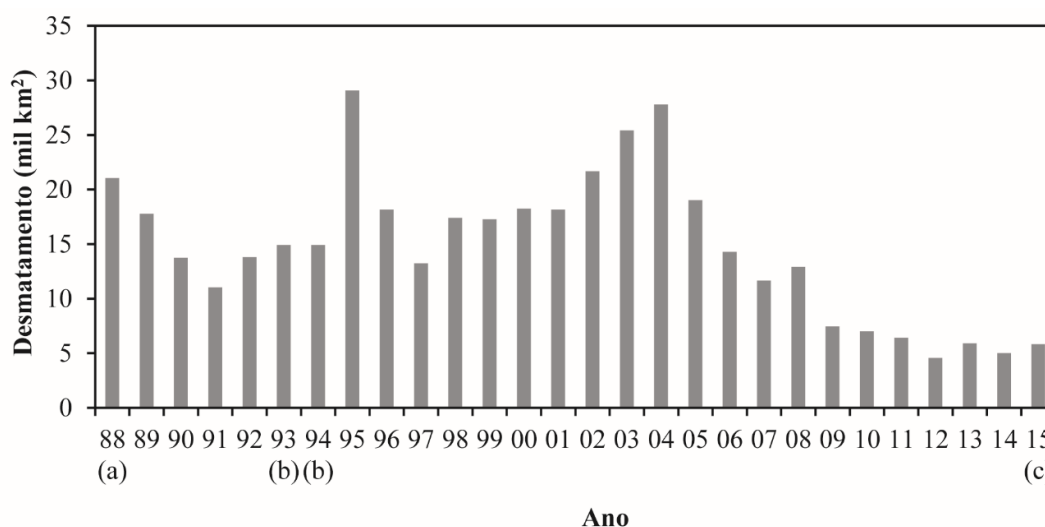
Figura 2.1 - Taxas de desmatamento na Amazônia Legal brasileira durante os anos de 1988 a 2015. (a) Média entre 1977 e 1988, (b) Média entre 1993 e 1994, e (c) Taxa estimada. Fonte: PRODES (2015).
