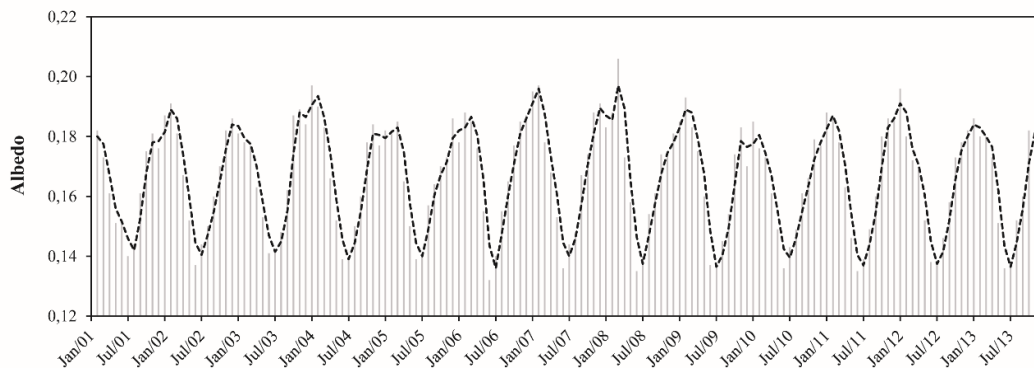
Figura 5.6 - Albedo mensal entre janeiro de 2001 e dezembro de 2013.
