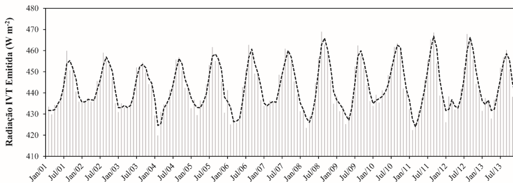
Figura 5.10 - Radiação IVT emitida mensal entre janeiro de 2001 e dezembro de 2013.
