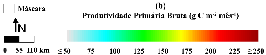
Figura 5.15 - Média anual (a) e médias mensais (b) de produtividade primária bruta considerando o período entre os anos de 2001 e 2013.
