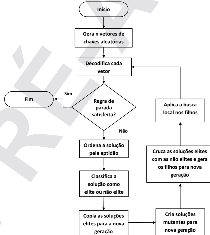
Figura 3: Fluxograma do BRKGA e heurística de busca local adaptada de Gonçalves e Resende [2011].
