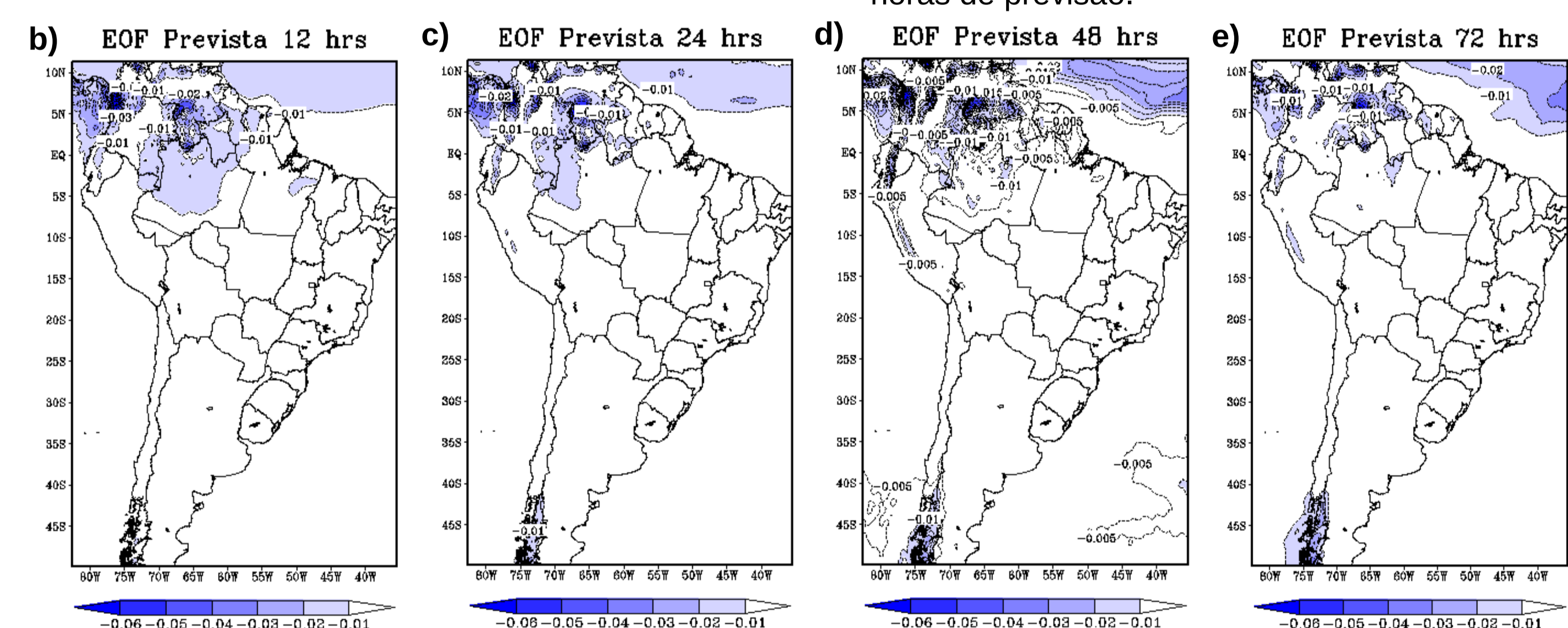
Figura 2 – Padrões de variabilidade obtidos com a primeira EOF calculada para os campos observados (a) e previstos pelo MCGA às 12 (b), 24 (c), 48 (d) e 72 (e) horas de previsão.
