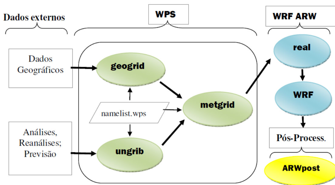
Figura 3.3: Representação esquemática do sistema de modelagem. Adaptado de ARW V3 Modeling System User's Guide , 2011.
