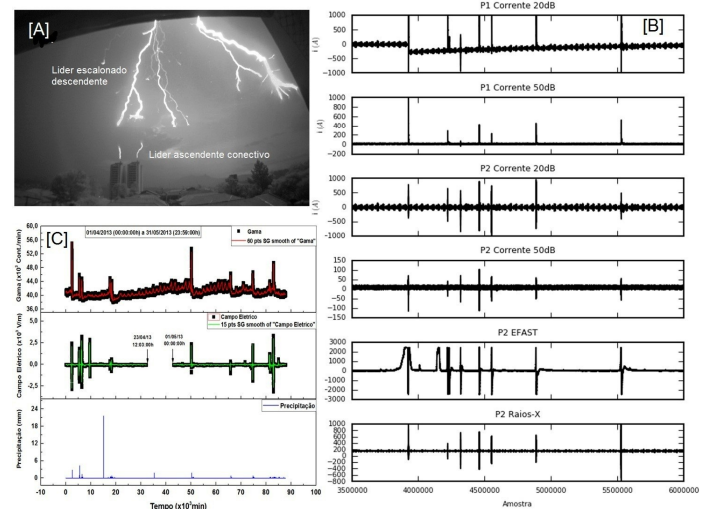
Figura 3 – [A] Líderes associados a um relâmpago nuvem-solo negativo.
