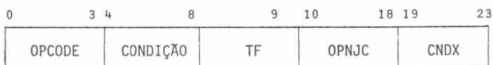
TIPO 3 - DESVIO CONDICIONAL
