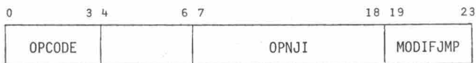
TIPO 4 - DESVIO INCONDICIONAL
