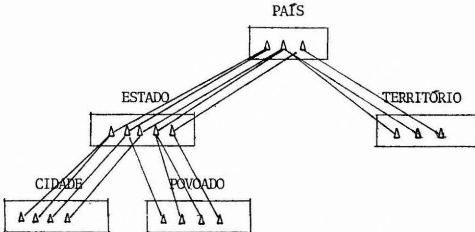
Fig. 5 - Banco de Dados Hierárquico.
