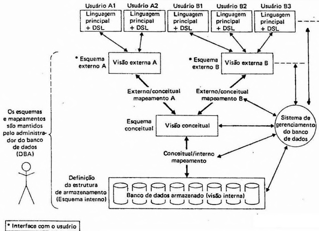
Fig. 3 - Arquitetura de um Banco de Dados.
