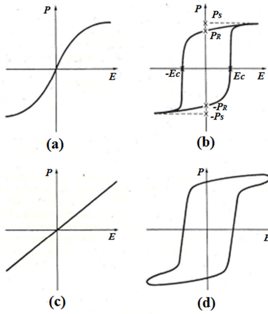
Figura 12- Curva P \times E (a) dielétrico não linear ideal, (b) dielétrico com perdas, (c) dielétrico linear e (d) dielétrico não linear com pobre contato elétrico dos eletrodos
