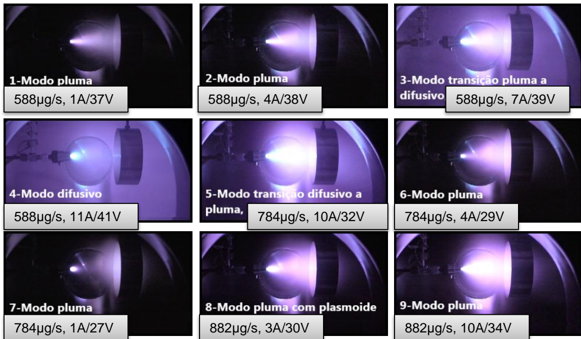
Figura 4.14- Sequência de variação dos modos de operação para diferentes correntes de descarga e vazões mássicas entre 588 e 882 \mu\text{g/s} , com gás xenônio para o catodo 10.
