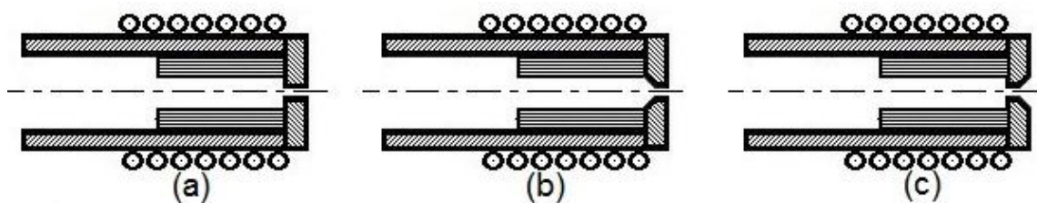
Figura 2.3- Tipos de orifício da ponteira do catodo oco: orifício cilíndrico (a), orifício convergente ou curvado (b) e orifício divergente (C).
