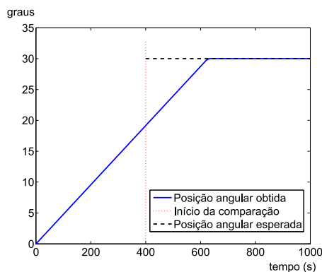
Figura 13: Apontamento para o sol esperado e obtido do satélite
