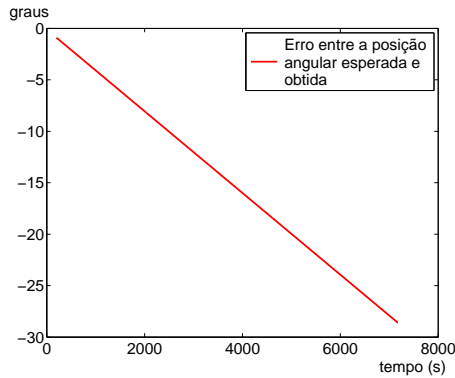
Figura 17: Erro de resposta à rampa de entrada no satélite
