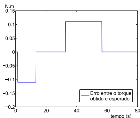
Figura 12: Erro computado no torque de saída da roda de reação
