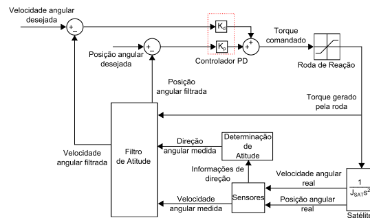
Figura 1: Modelo de sistema de controle simplifi- cado de um satélite
