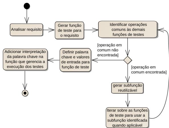
Figura 4: Atividade que processa um requisito para gerar a função de teste
