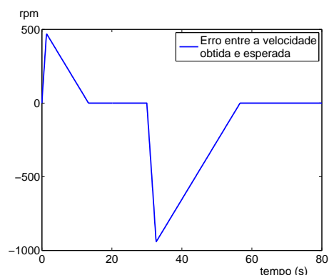
Figura 10: Erro computado na velocidade da roda de reação
