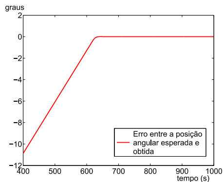
Figura 14: Erro de apontamento para o Sol do satélite
