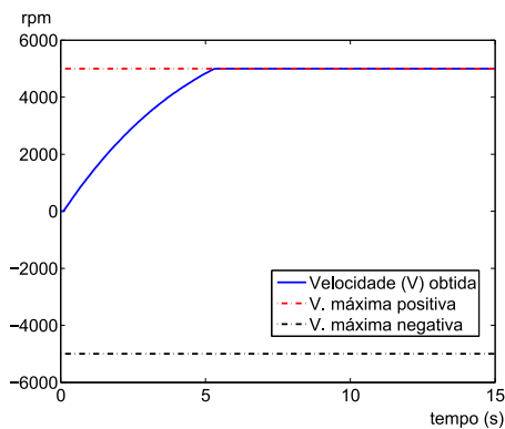
Figura 18: Velocidade gerada pela roda de reação em malha fechada (entrada rampa)
