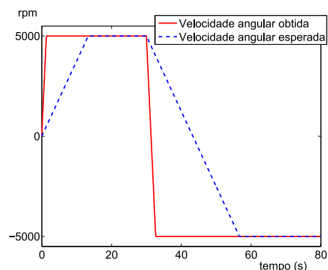
Figura 9: Velocidade esperada e obtida da roda de reação
