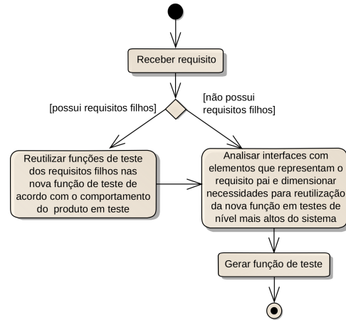
Figura 3: Geração de função de teste para um requisito específico
