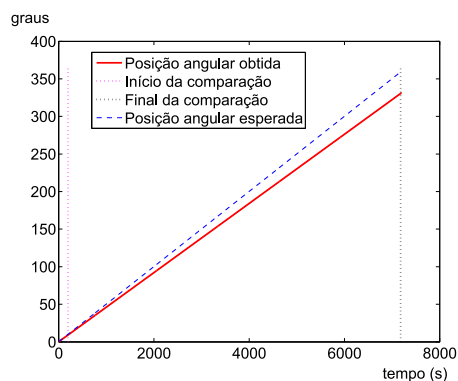
Figura 16: Apontamento (sinal rampa) esperado e obtido do satélite
