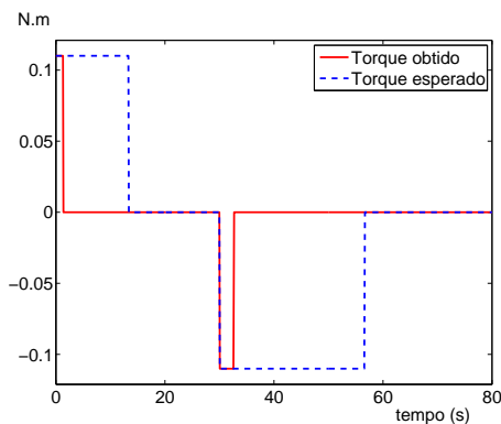
Figura 11: Torque esperado e obtido da roda de reação
