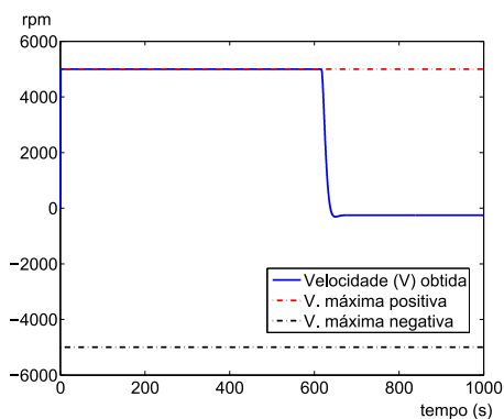
Figura 15: Velocidade gerada pela roda de reação em malha fechada (apontamento para o Sol)
