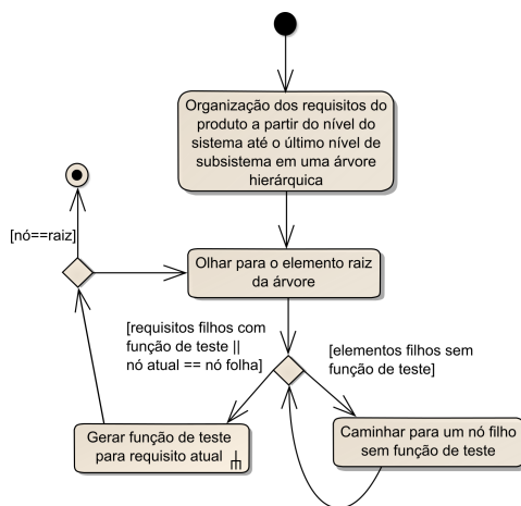
Figura 2: Descrição da mecânica para a geração das funções de teste para o sistema
