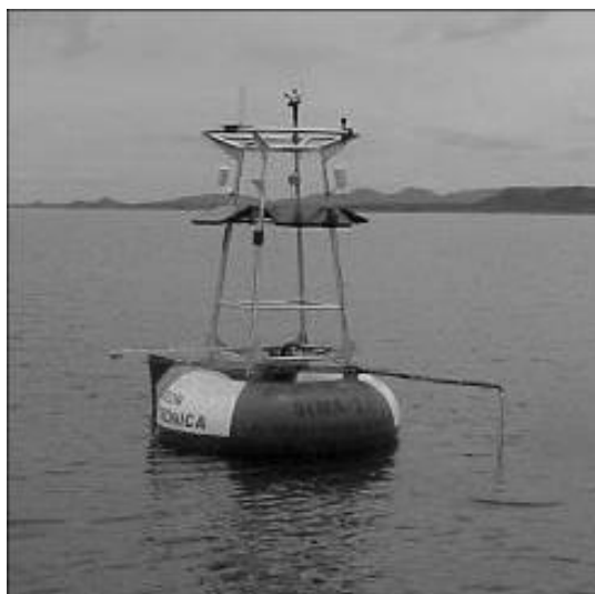
Figura 7.8 – SIMA instalado no reservatório de Serra da Mesa
