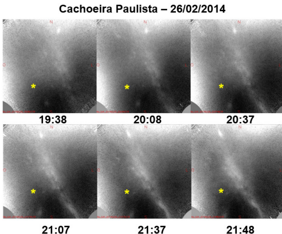
Figura 4.15 - Sequência de imagens de airglow da emissão de sódio em 26 de fevereiro de 2014.
