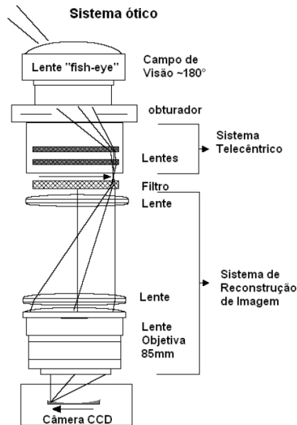
Figura 3.9 - Sistema óptico do imageador all-sky instalado em Cachoeira Paulista. FONTE: Wrasse, 2004.
