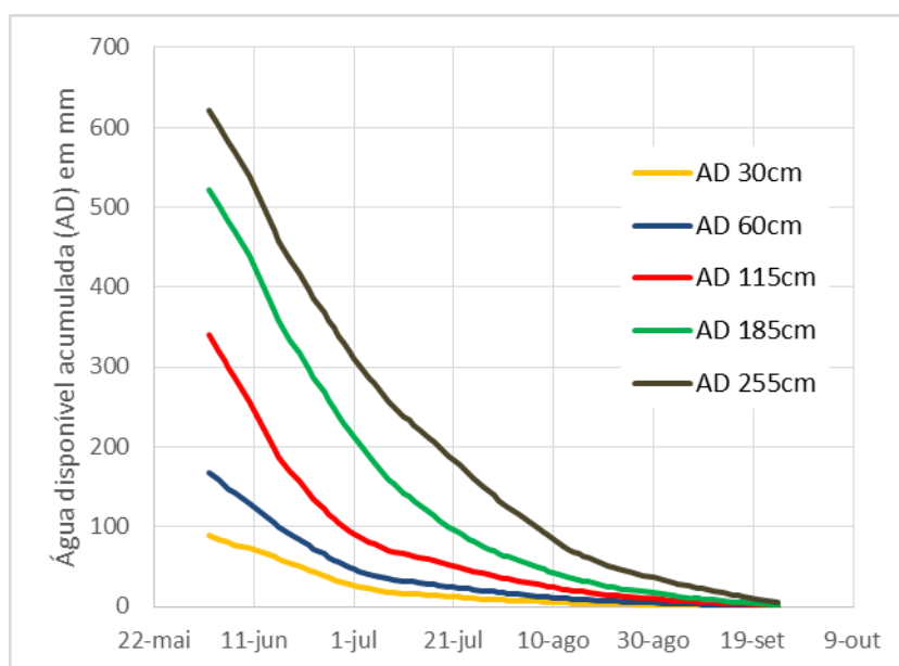
Figura 4.7 – Evolução temporal da água disponível acumulada ( AD ).
