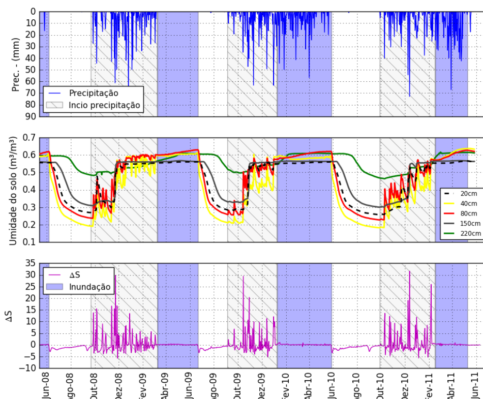
Figura 4.1 – Valores de precipitação diária (mm), médias diárias de umidade volumétrica do solo ( \theta , em \text{m}^3 \cdot \text{m}^{-3} ) para as profundidades de 20, 40, 80, 150 e 220 e a taxa de variação de água do solo \Delta S ( \text{mm} \cdot \text{dia}^{-1} ). As barras azuis indicam o período de inundação onde \Delta S é próximo de 0. As barras hachuradas indicam o período de início de precipitação onde \Delta S apresenta grande variação.
