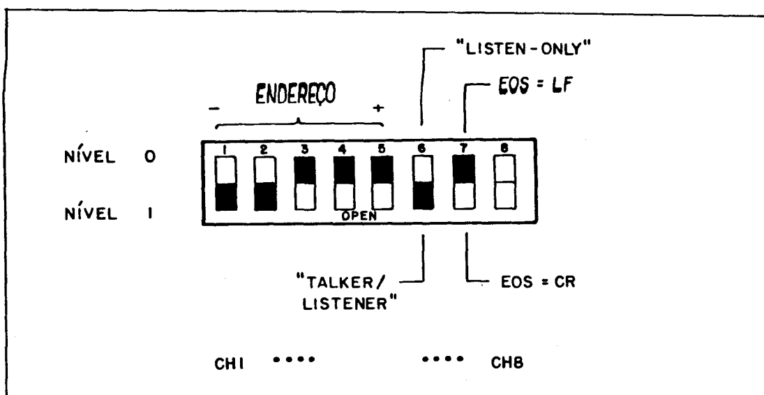
Fig. 8 - Chaves para operação via GPIB.
