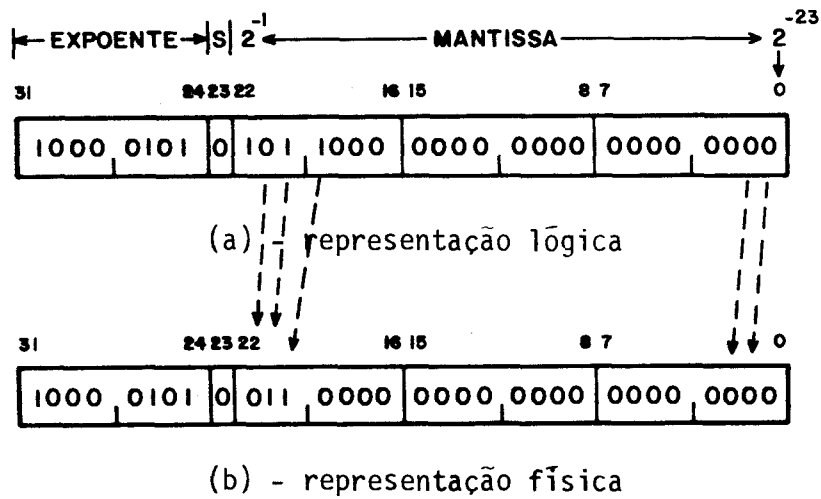
Fig. 3.2 - Representação em ponto flutuante.
